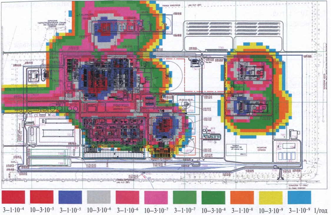
Рис. 7-2. Территориальное распределение превышения избыточного давления во фронте УВ (120 кПа) для сценариев Впво на объекте
