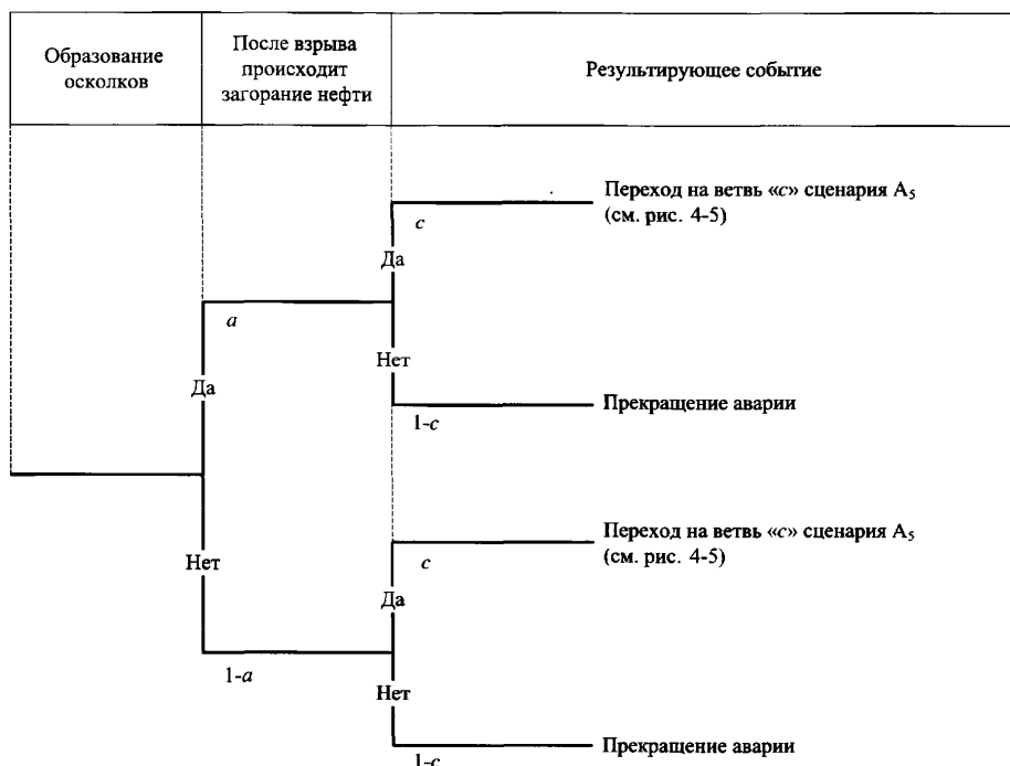
Рис. 4-6. Дерево событий при взрыве внутри подземного резервуара (типа ЖБР) (сценарий A_6 )
