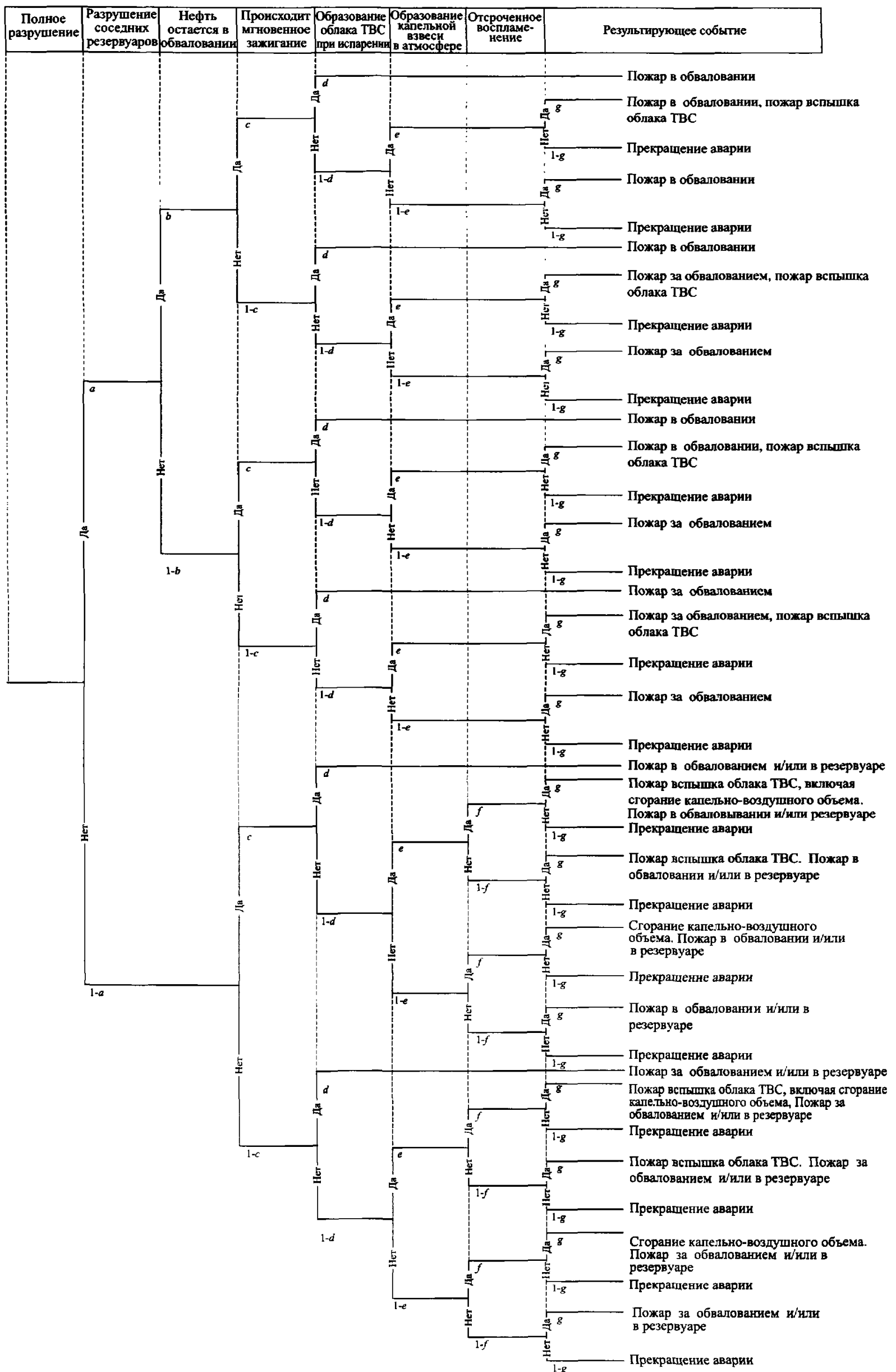
Рис. 4-1. «Дерево событий» разрушения/перелива наземного резервуара (сценарий А 1 )
