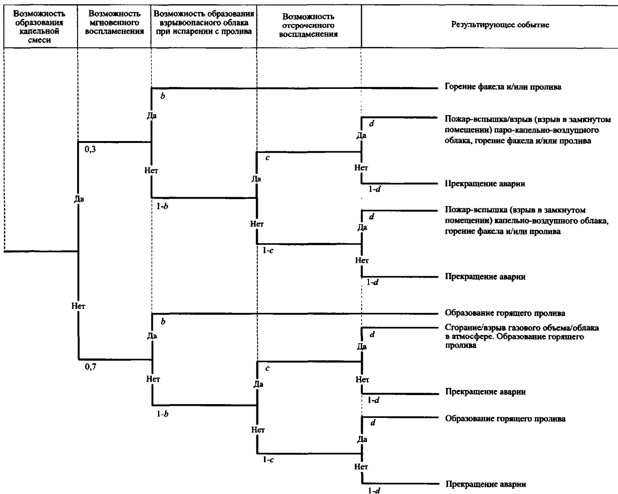
Рис. 4-9. Дерево событий при аварии в насосных (сценарий A 9 )
