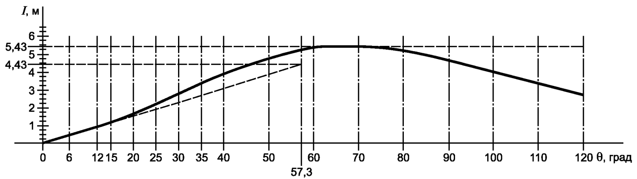
Рисунок К.12 — Диаграмма статической остойчивости
