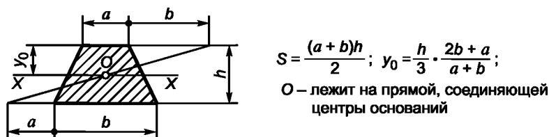
Рисунок К.5 — Определение площади и центра тяжести трапеции
