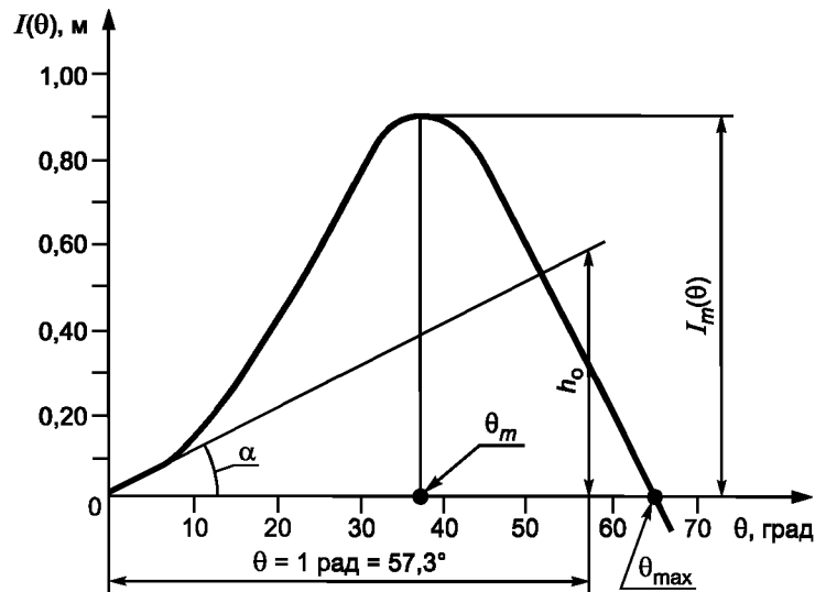
Рисунок К.3 — Диаграмма статической остойчивости
