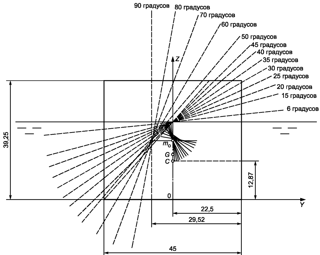
Рисунок К.8 — Положения ватерлиний и соответствующих им перпендикуляров при изменении углов крена от 0° до 90°
