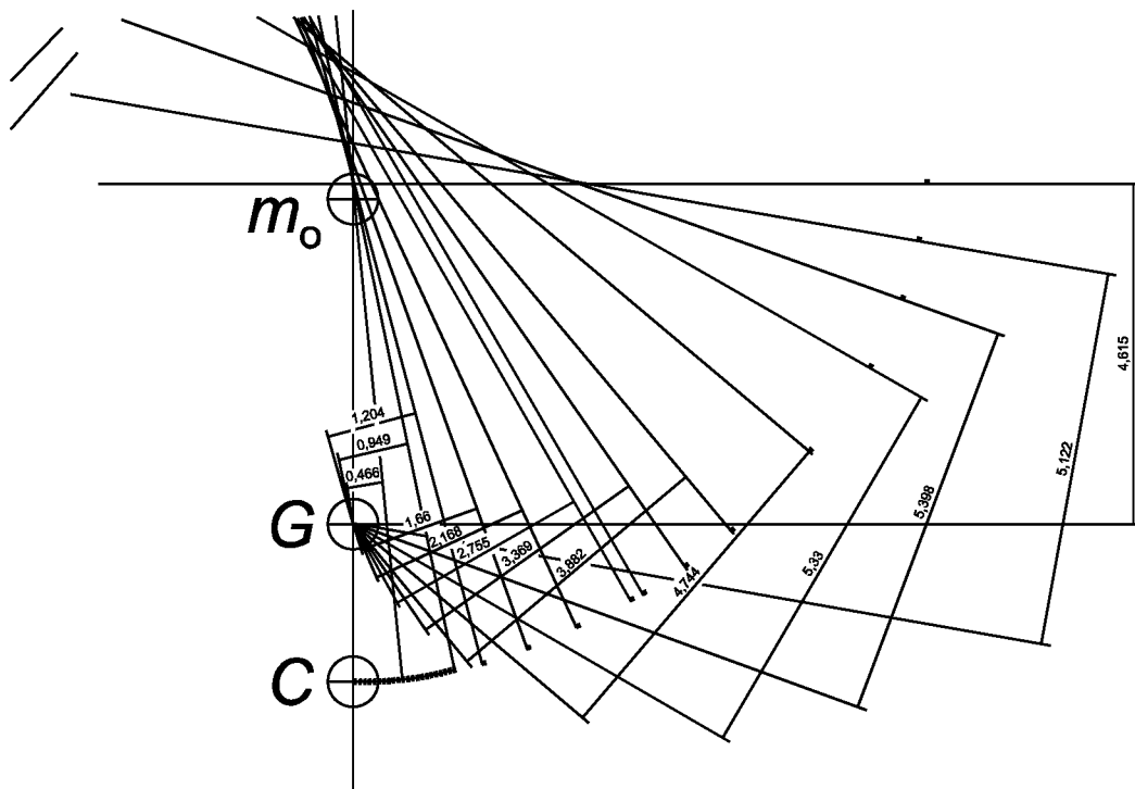
Рисунок К.9 — Измеренные плечи пар сил I(\theta)_l при кренах от 0° до 90°
