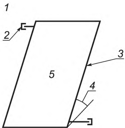
1 — Водные брызги на всех сторонах; 2 — Трубопровод, запечатанный с накидной гайкой; 3 — Нижняя сторона коллектора, защищенная для коллекторов, разработанных для интеграции в конструкцию крыши; 4 — Угол наклона; 5 — Коллектор
