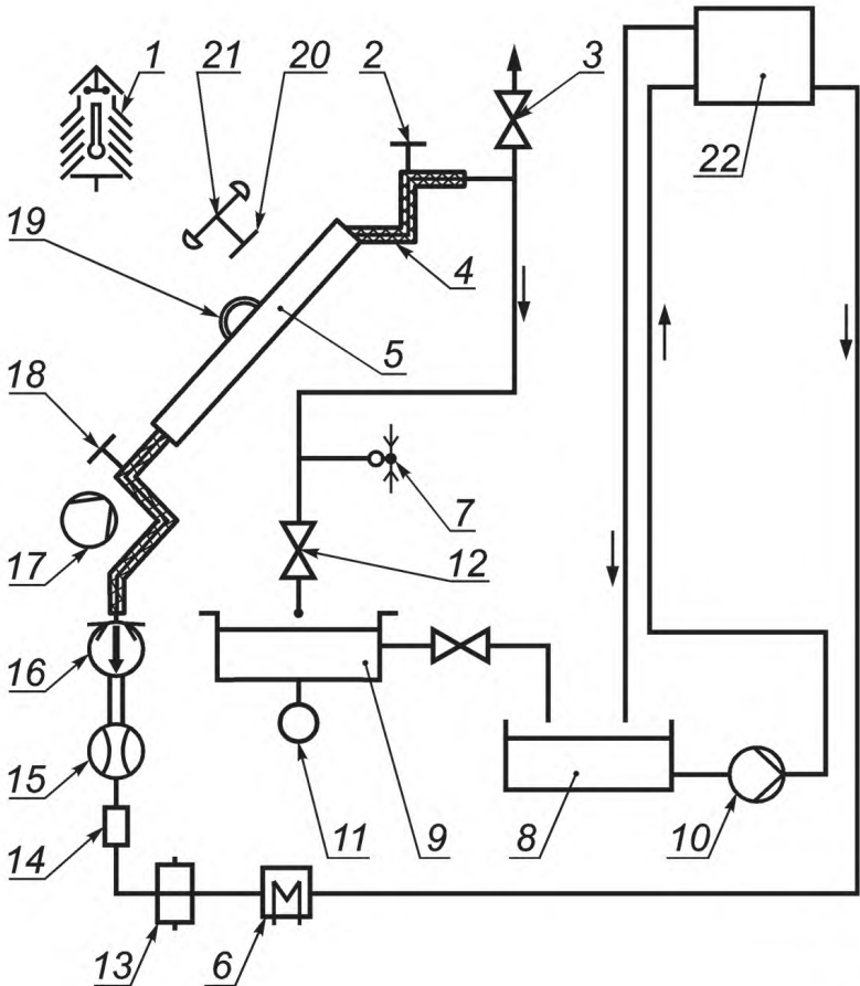
Рисунок 3 — Пример открытого (разомкнутого) испытательного контура
