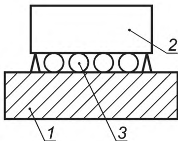
1 — Жесткая поддержка; 2 — Коллектор; 3 — Воздушные подушки, чтобы применить давление
