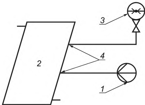
1 — Источник пневматического давления; 2 — Коллектор; 3 — Манометр; 4 — Отверстия в зазоре между покрытием коллектора и поглотителем
