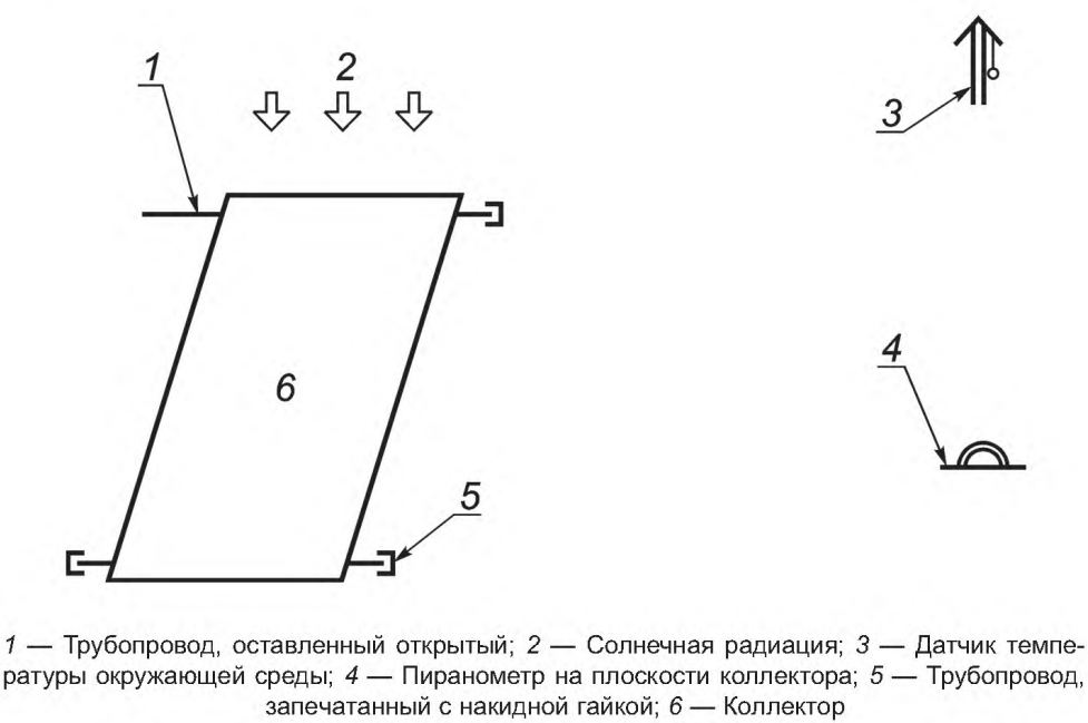
Рисунок А.7 — Описание схемы для испытания на воздействие атмосферных условий
