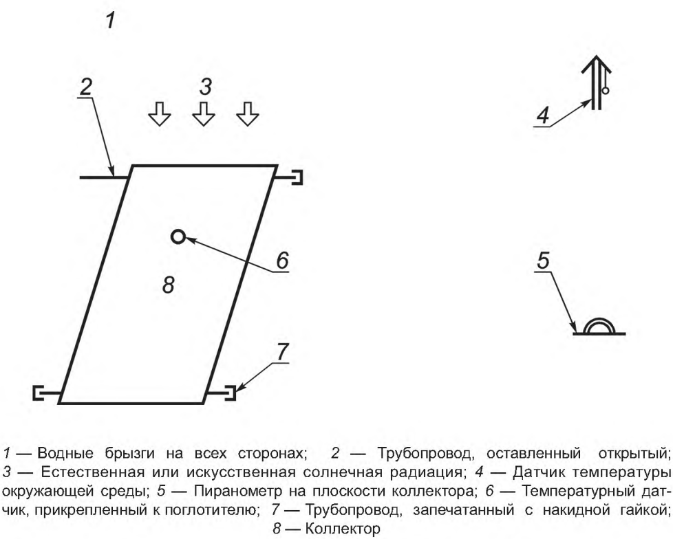
Рисунок А.8 — Описание схемы для испытания на внешний тепловой удар
