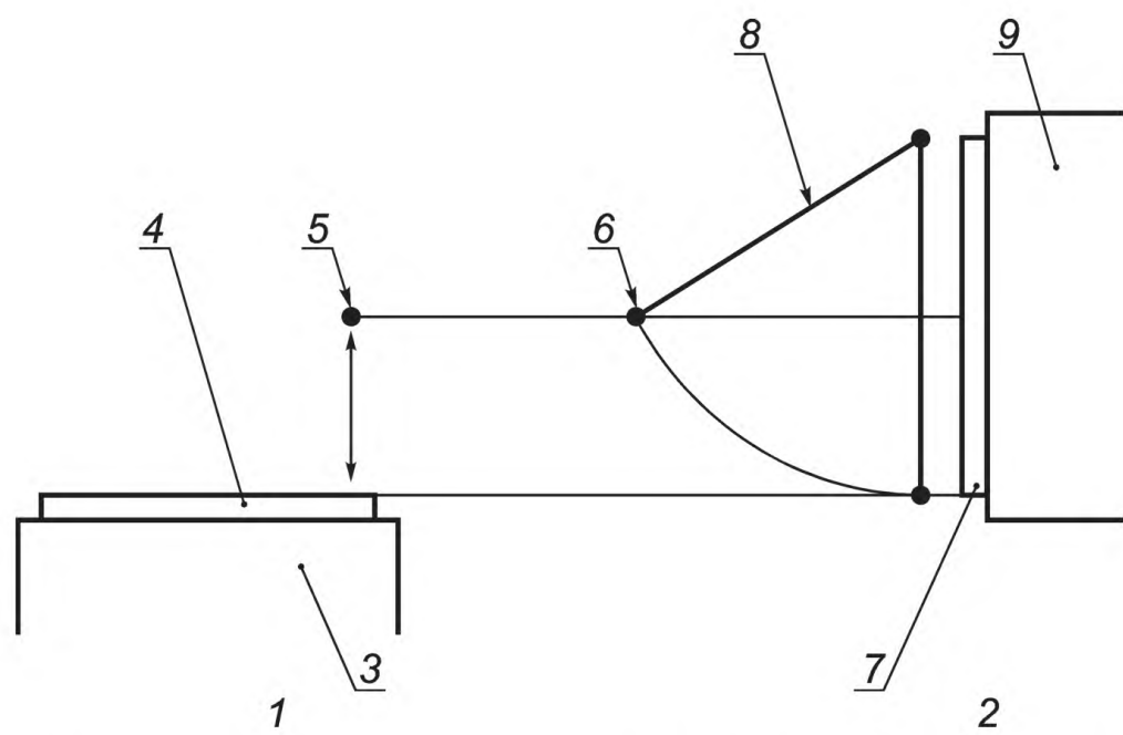
1 — Альтернатива А (стальной шар, падающий вертикально); 2 — Альтернатива В (маятник); 3 — Жесткая рама; 4 — Коллектор; 5 — Стальной шар; 6 — Стальной шар; 7 — Коллектор; 8 — Маятник; 9 — Жесткая рама
