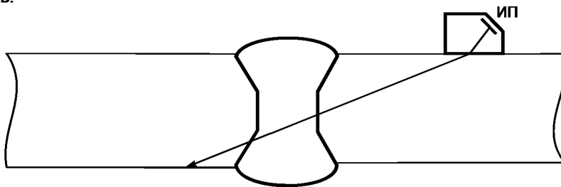
Рисунок 7 — Схема прозвучивания стыкового сварного соединения прямым лучом
