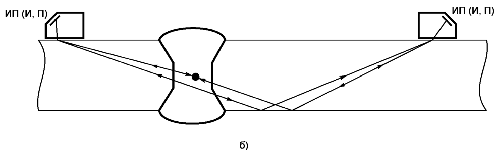
Рисунок 3 — Эхо-теневого прямым (а) и наклонными (б) ПЭП
