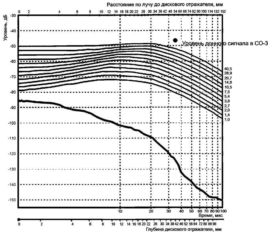
РШХ без акустической нагрузки и АРД-диаграмма
