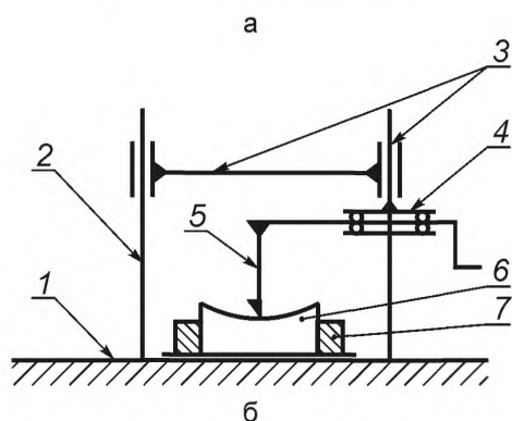
1 — основание прибора; 2 — стойка; 3 — звенья для перемещения резца; 4 — приспособление для закрепления и вращения резца; 5 — резец; 6 — образец (деталь); 7 — устройство для закрепления образца (детали)
