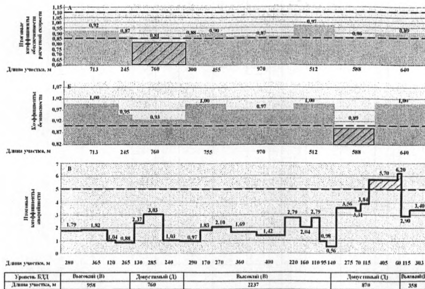
Рисунок Б. 1 – Пример оценки уровня безопасности дорожного движения на участке двухполосной дороги на стадии подготовки инженерного проекта
