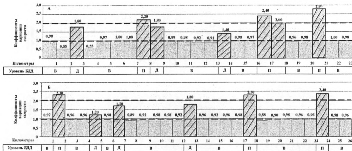
Рисунок Б. 3 – Пример оценки качества вариантов проектов нового строительства на стадии подготовки проекта планировки территории для размещения автомобильной дороги категории IB
