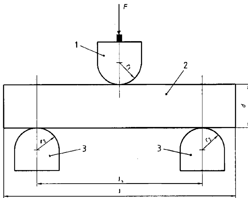
1 – нагрузка; 2 – образец; 3 – опора l – длина образца; d – диаметр образца; l_s – расстояние между опорами; r_1, r_2 – радиусы опор
