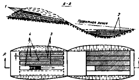
1 – ярусы; 2 – слой отсыпанной насыпи; 3 – траншеи яруса; 4 – стенки
