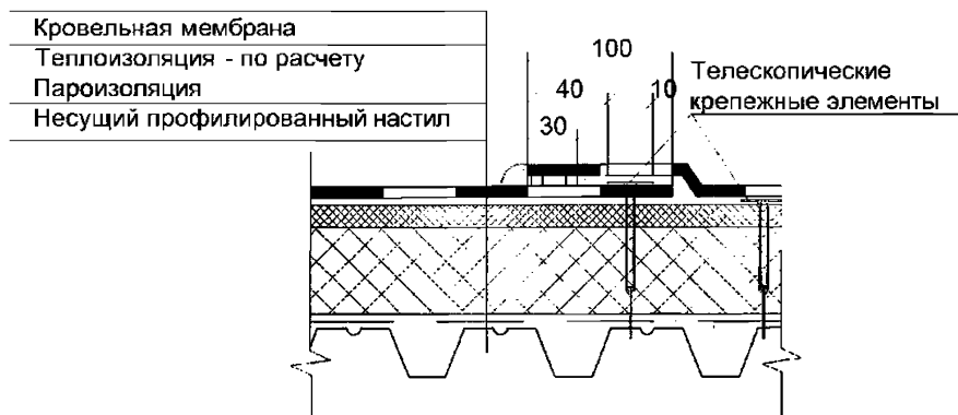
Рисунок 3 – Механическое крепление мембраны, уложенной на утеплитель
