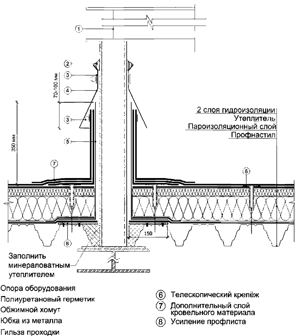
Рисунок 1 – Устройство примыкания к опоре с гильзой на плоской крыше
