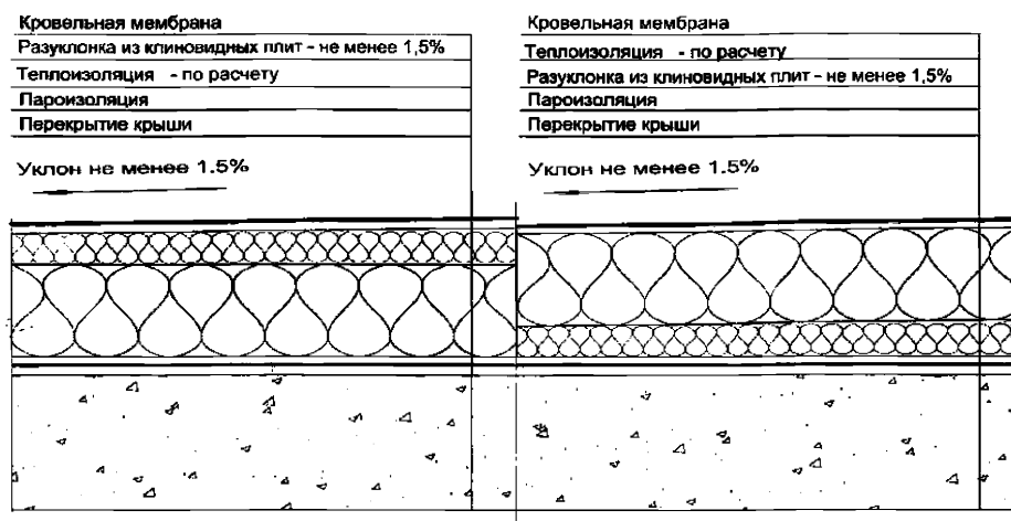
Рисунок 2 – Варианты уклонообразующего слоя из ТМ
