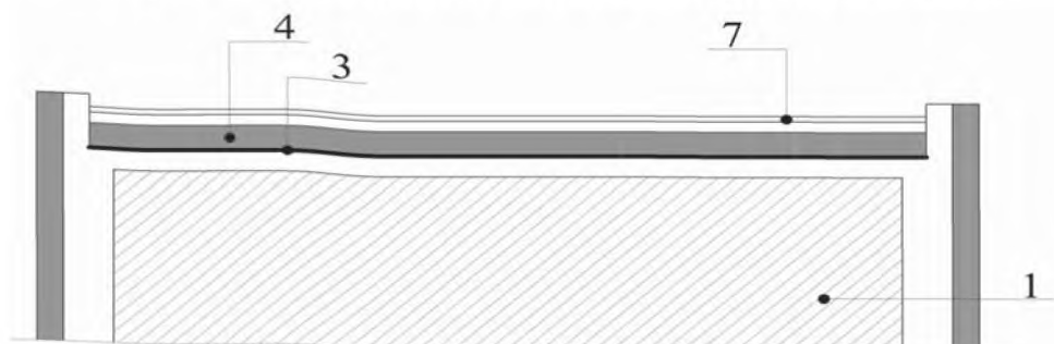
г – утепленная совмещенная плоская крыша
