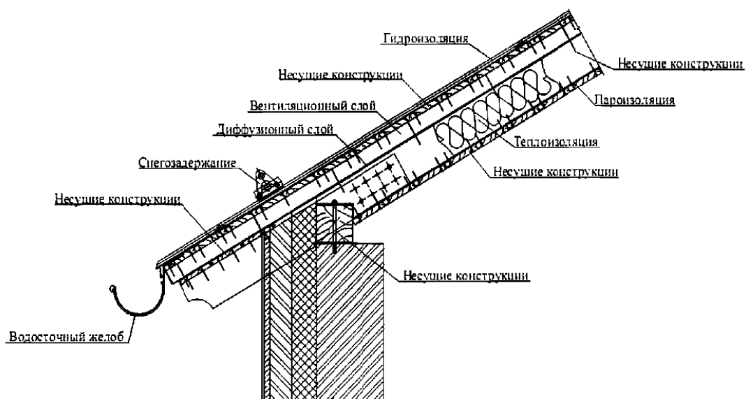
Рисунок А.1 – Слои скатной крыши
