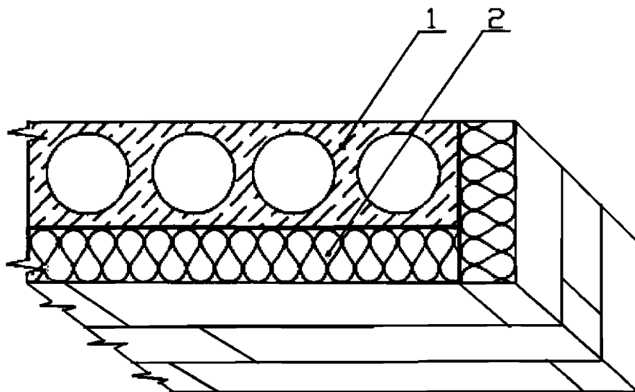
Рисунок 6.8 – Пример выполнения зубчатого зацепления плит
