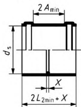
Рисунок 7 – Муфта
