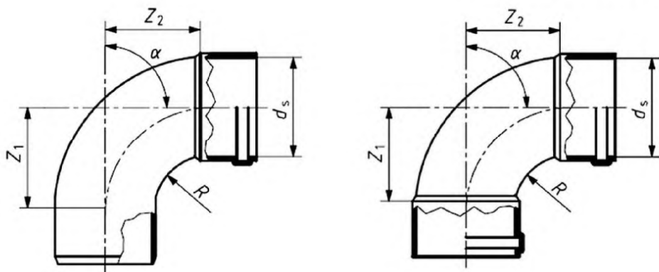
Рисунок 6 – Отвод
