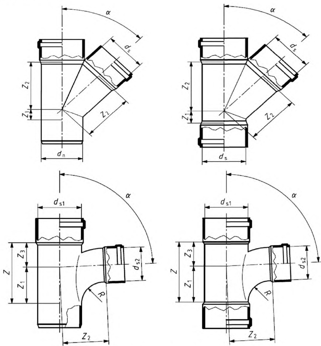
Рисунок 9 – Тройник
