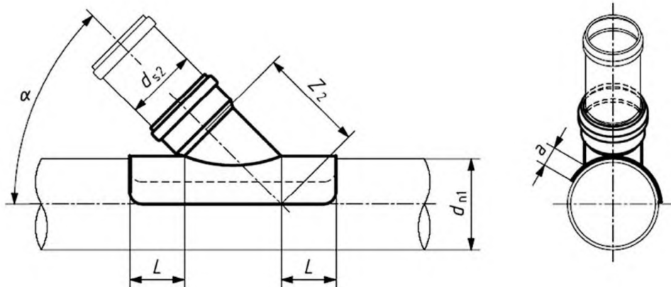
Рисунок 10 – Седловой отвод
