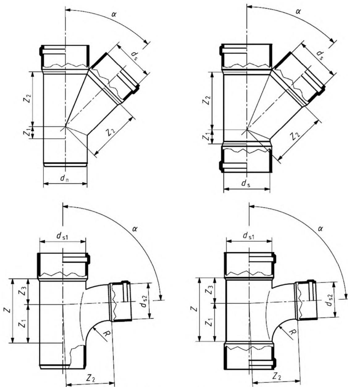
Рисунок 9 – Тройник
