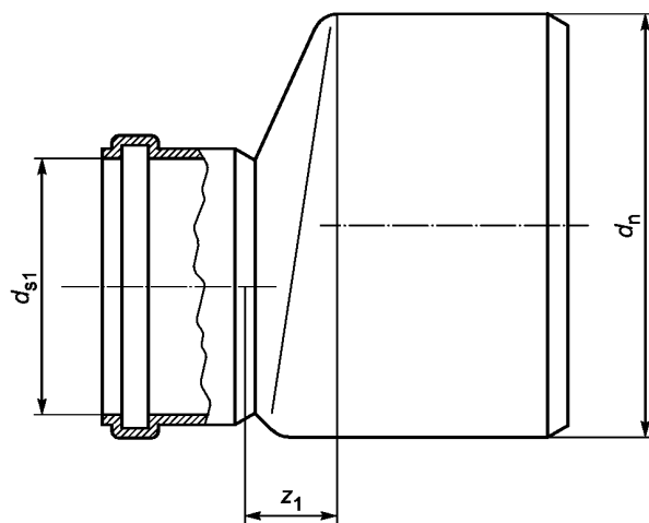
Рисунок 7 — Патрубок переходной
