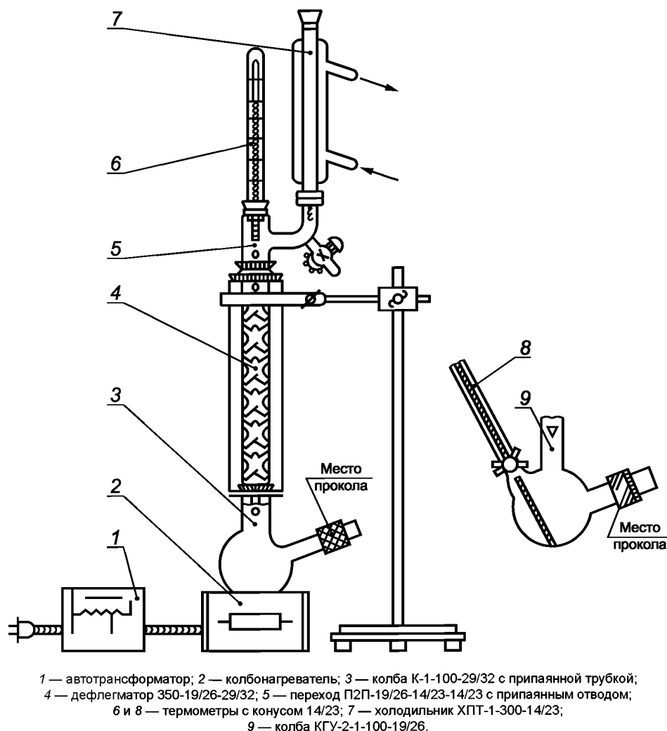
Рисунок 2 — Установка для определения массовой доли пропеллента
