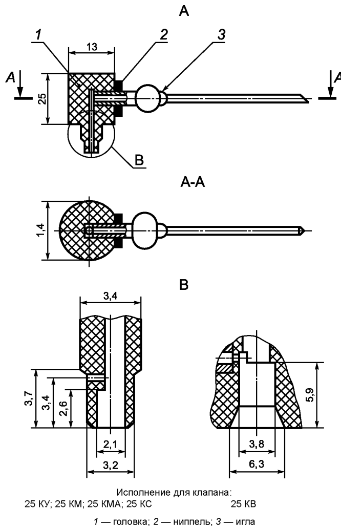
Рисунок 1 — Распылительная головка с инъекционной иглой
