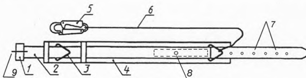
1 – пряжка; 2 – ремень; 3 – боковое кольцо; 4 – кушак; 5 – карабин; 6 – фал; 7 – люверсы; 8 – амортизатор с чехлом и контрольным люверсом; 9 – шпенец
