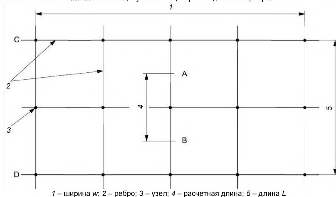
Рисунок 7 – Стандартная георешетка
