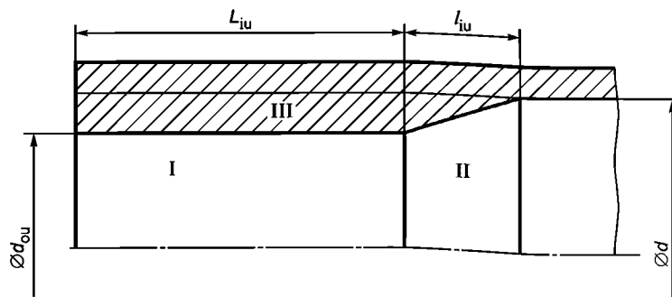
Рисунок 10 — Внутренняя высадка
