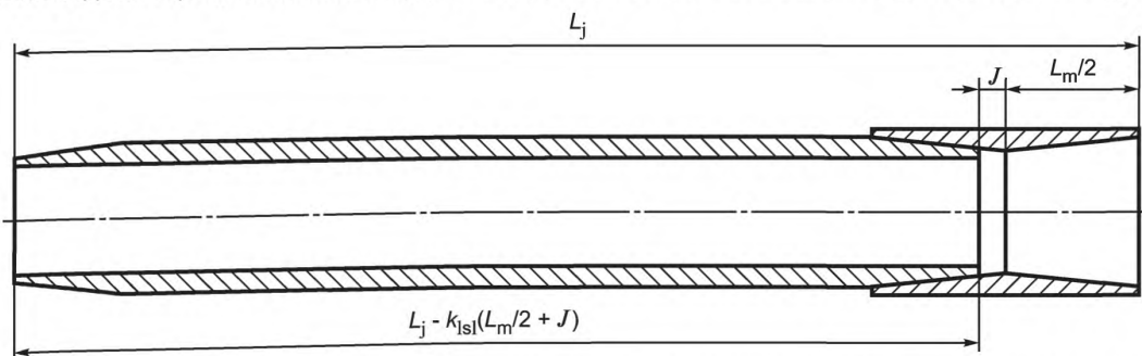
Рисунок 2 — Труба с резьбой и муфтой
