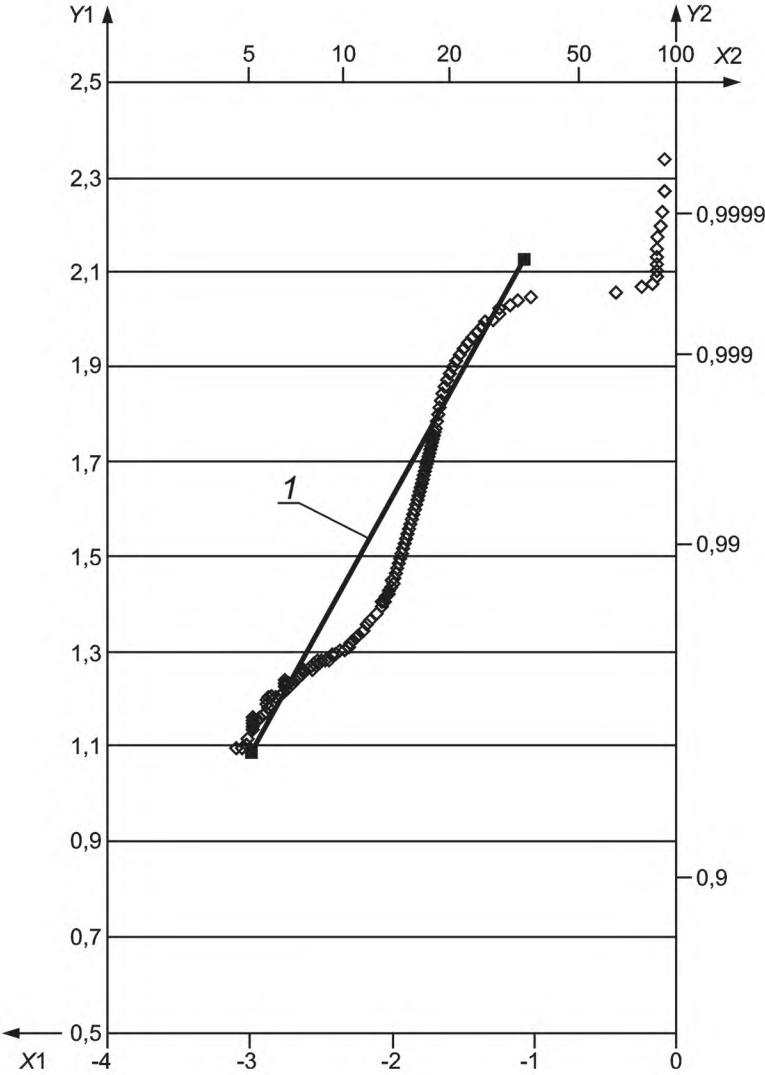
1 — прямая Вейбулла при параметре b , равном 0,55
