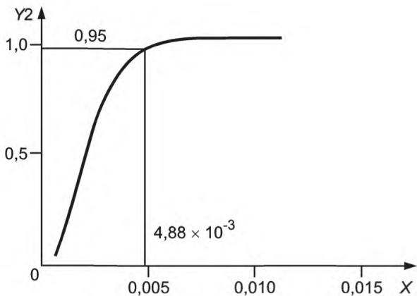
б — Функция кумулятивного распределения CDF
