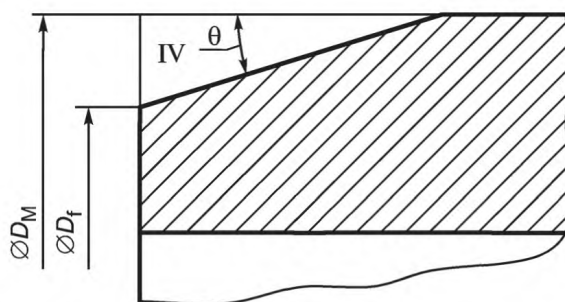
Рисунок 4 — Муфта с треугольной резьбой
