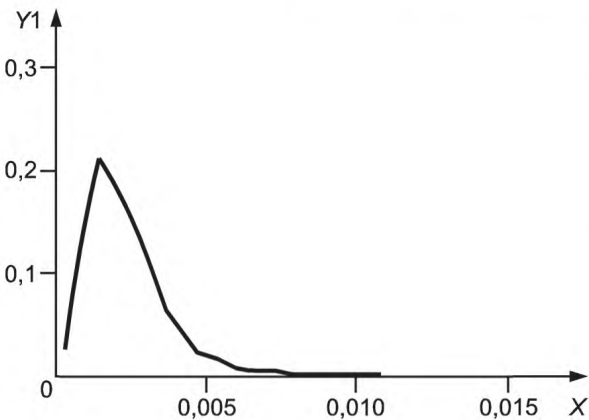
а — Функция распределения вероятностей PDF
