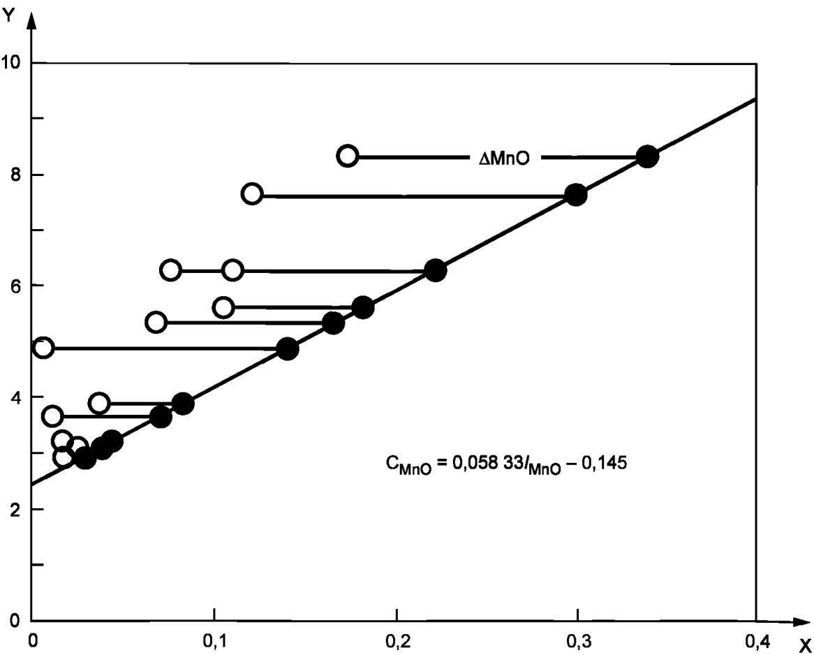
по оси X — C_{MnO} , % по оси Y — интенсивность рентгеновского излучения ( I ) линии Mn K \alpha \Delta MnO в процентах от массы MnO показывает разницу между измеренным значением (белые точки) и расчетным (черные точки) на предполагаемой основной калибровочной кривой для Cr_2O_3 , не содержащего MnO.
