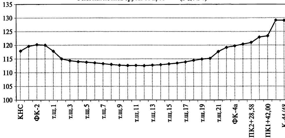
Отметки лотков трубы от н/ст **** (в-д № 1)
