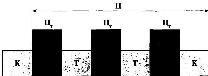
Рис. 1. Структурная схема ремонтного цикла
