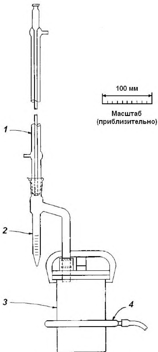
1 – холодильник; 2 – приемник; 3 – металлический перегонный куб; 4 – кольцевая горелка П р и м е ч а н и е – Приемник должен иметь внутренний диаметр от 15 до 16 мм. Рисунок 3 – Типичная сборка с металлическим перегонным кубом
