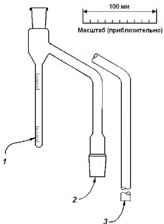
1 – интервал градуировки – 0,05 \text{ см}^3 ; 2 – конусное соединение; 3 – простое соединение Рисунок 2 – Приемник с различными соединениями к стеклянному перегородочному кубу вместимостью 2 \text{ см}^3
