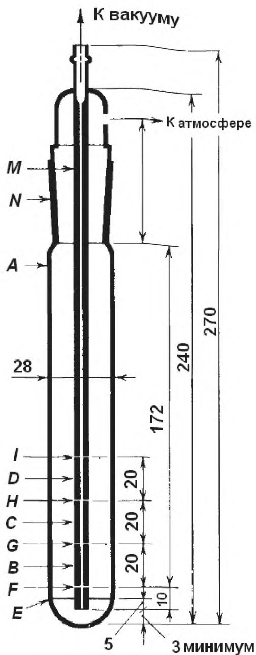
Рисунок 4 – Модифицированный вакуумный вискозиметр Копперса (МКВВ)
