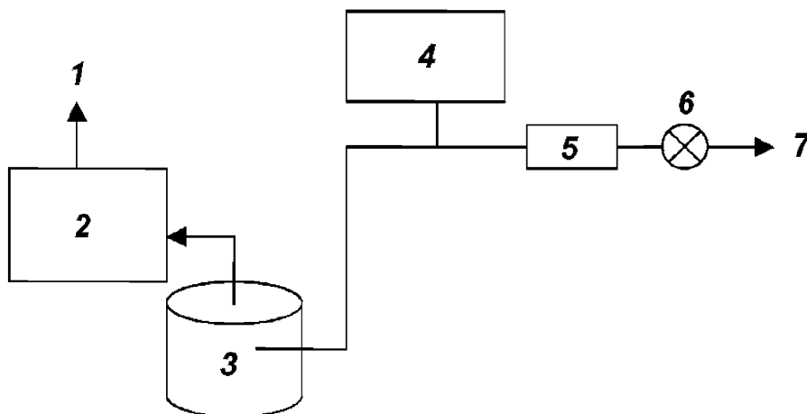
1 – к вакуумному насосу; 2 – система контроля давления; 3 – буферный резервуар вместимостью 1 дм 3 ; 4 – манометр; 5 – ловушка; 6 – переключающий кран; 7 – к вискозиметру Рисунок 1 – Схема вакуумной системы для вакуумных капиллярных вискозиметров
