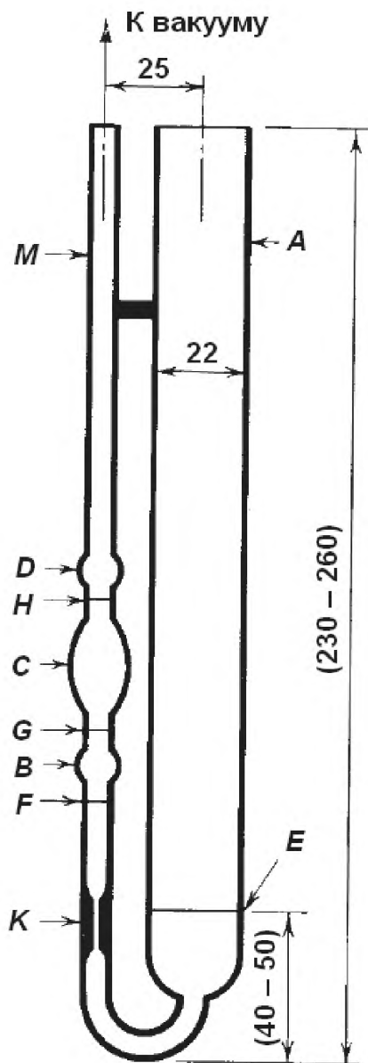
А – трубка заполнения; В, С, D – шарики; Е – линия заполнения; F – первая метка времени; G – вторая метка времени; H – третья метка времени; K – капилляр; M – вакуумная трубка Рисунок 2 – Вакуумный вискозиметр Кэннон-Мэннинга (CMVV)
