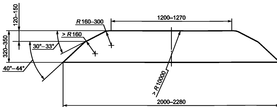
Рисунок 1 — Конфигурация и размеры ползов
