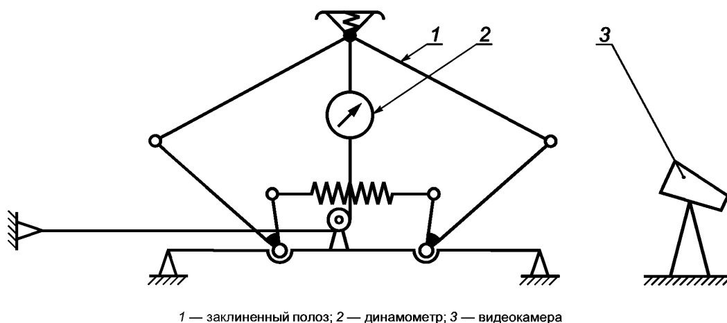
Рисунок 10 — Схема для определения вертикальной составляющей аэродинамической силы
