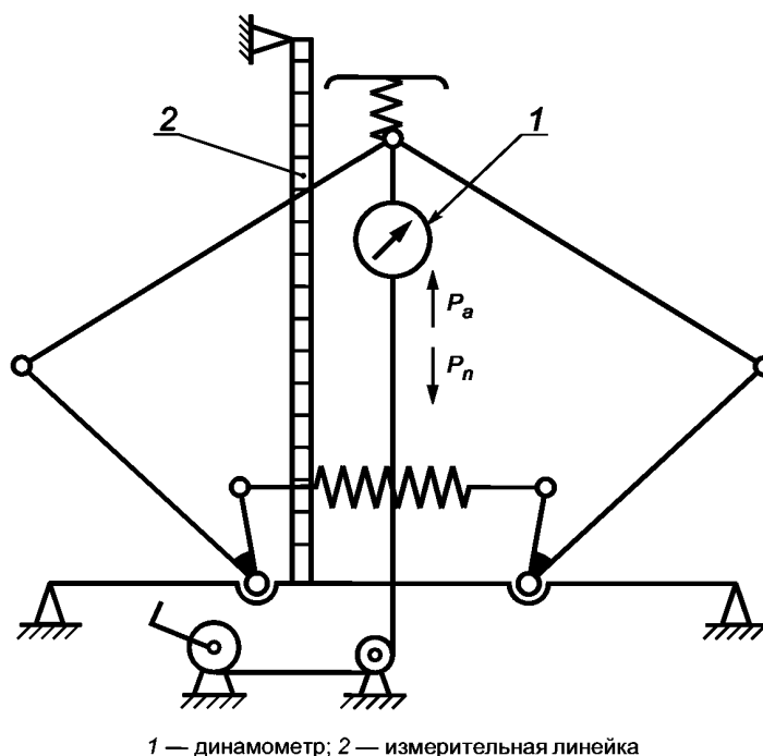
Рисунок 2 — Кинематическая схема для снятия статической характеристики
