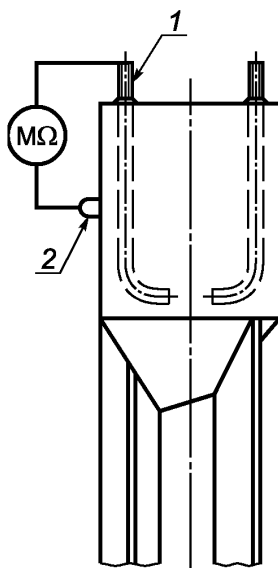
1 — болт анкерный; 2 — петля страховочная
