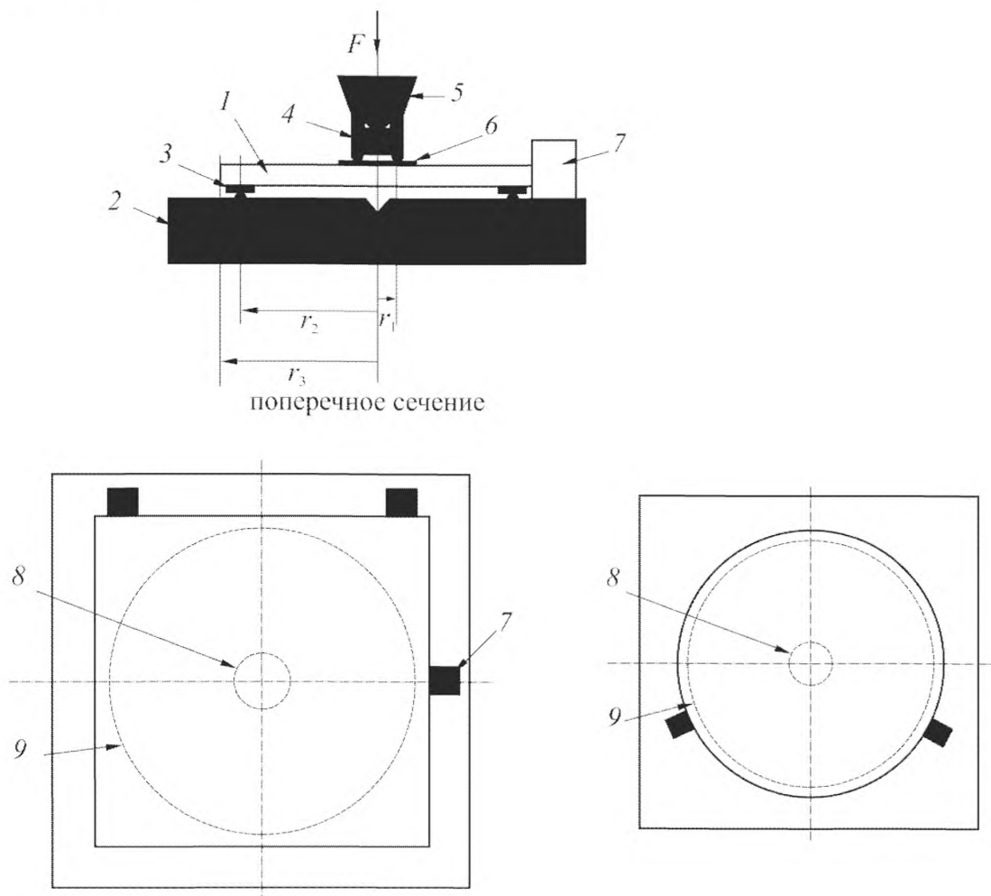
квадратный образец круглый образец 1 – образец; 2 – опорная плита из закаленной стали, снабженная опорным кольцом; 3 – прокладка из силиконовой резины; 4 – нагружающее кольцо из закаленной стали; 5 – передающий нагрузку элемент с центровкой для нагружающего кольца; 6 – прокладка из бумаги или синтетического материала толщиной приблизительно 0,1 мм; 7 – корректирующий упор для центровки образца; 8 – окружность контакта нагружающего кольца; 9 – окружность контакта опорного кольца
