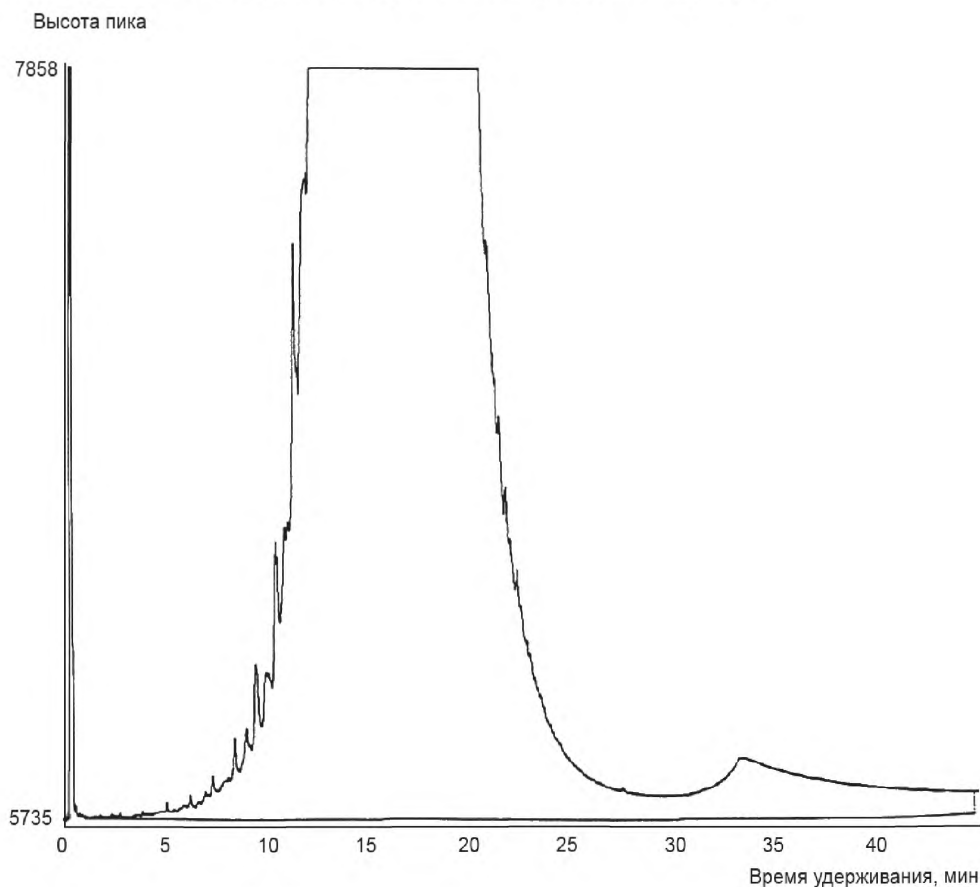
Рисунок 2 – Определение базовой линии образца моторного масла
