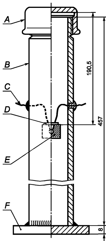
А — кованный стальной колпак; В — стальная труба; С — выводы воспламенителя; D — уплотнение; E — комплект воспламенителя; F — контрольная плита
