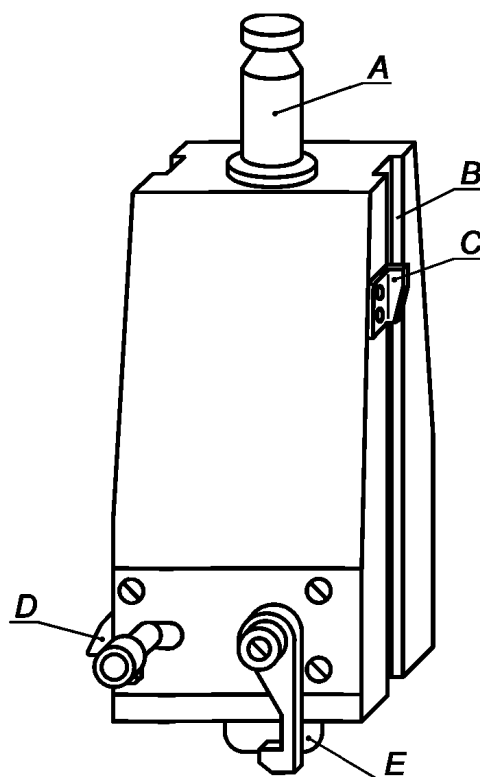
Рисунок 13 — Падающий груз
