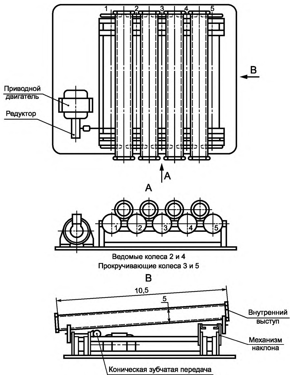
Рисунок 3 — Вращающиеся трубы
