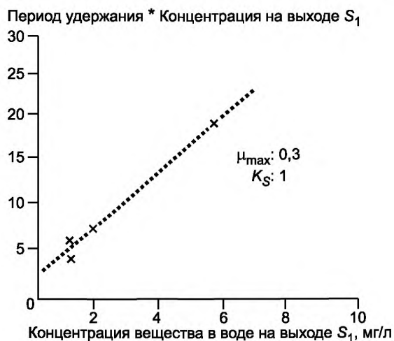
Рисунок Д.2 — Линия регрессии, период удержания S_1 от S_1 , T = 5^\circ\text{C}
