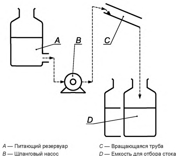
Рисунок 4 — Технологическая схема
