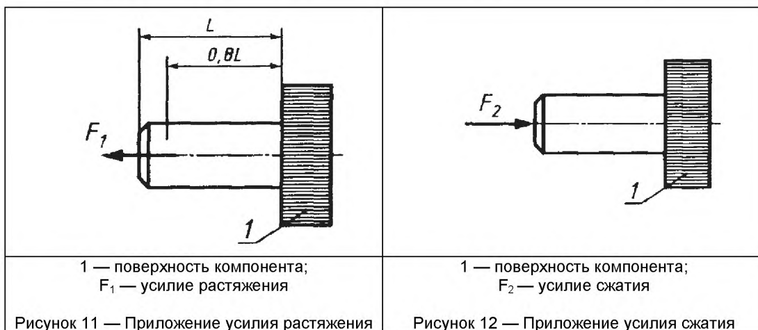
Рисунок 11 — Приложение усилия растяжения
