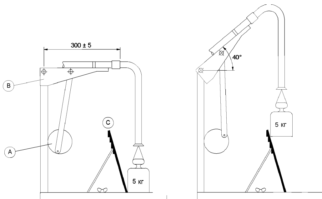
А – кривошипный механизм; В – рычаг; С – наклонная плоскость
