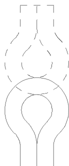
Положение шланга в начале и конце каждого изгиба Рисунок 104 – Положения изгиба для шланга после извлечения из морозильного шкафа
