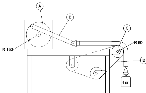
А – кривошипный механизм; В – соединительная тяга; С – ролик диаметром 120 мм; D – ремень с абразивной лентой
