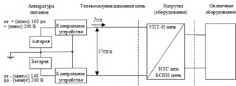
Рисунок 2 – Пример УПТ-Н системы удаленного электропитания
