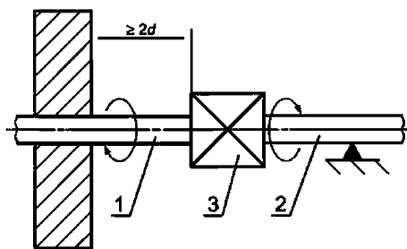
d – наружный диаметр; 1 – труба; 2 – труба; 3 – испытуемый образец
