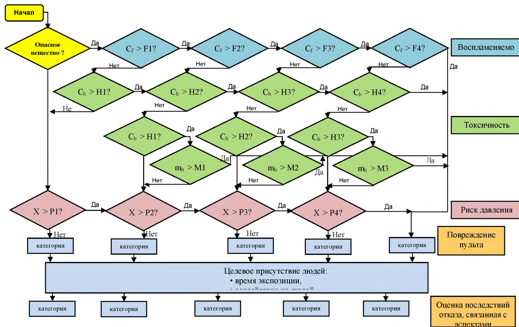
Рисунок 9 – Пример оценки последствий отказа, связанного с обеспечением безопасности ( X = P_w V + \frac{mT^2}{32000} )
