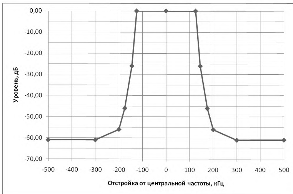
Рисунок 3 – Маска огибающей внеполосных радиопомех для ширины полосы частот 250 кГц
