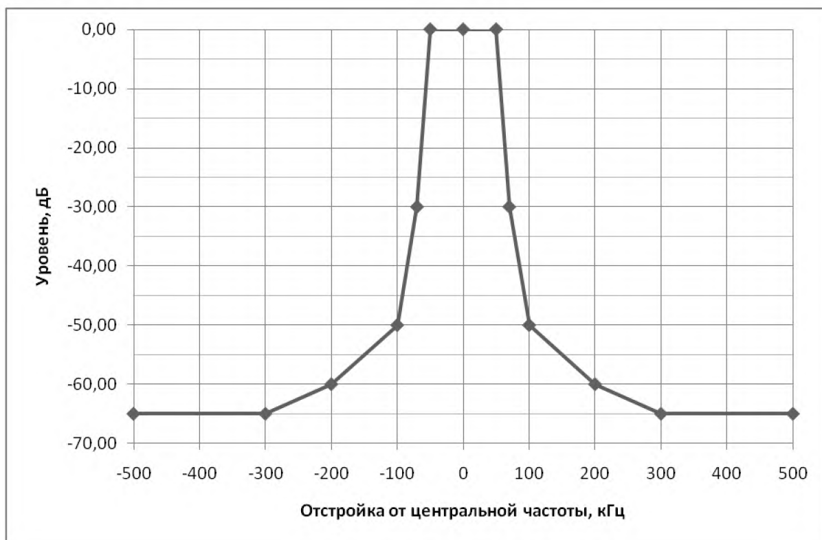
Рисунок 1 – Маска огибающей внеполосных радиополебаний для ширины полосы частот 100 кГц
