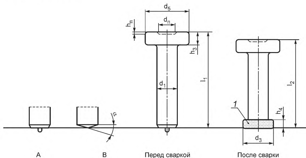
Рисунок 5 — Шпилька-упор (SD)
