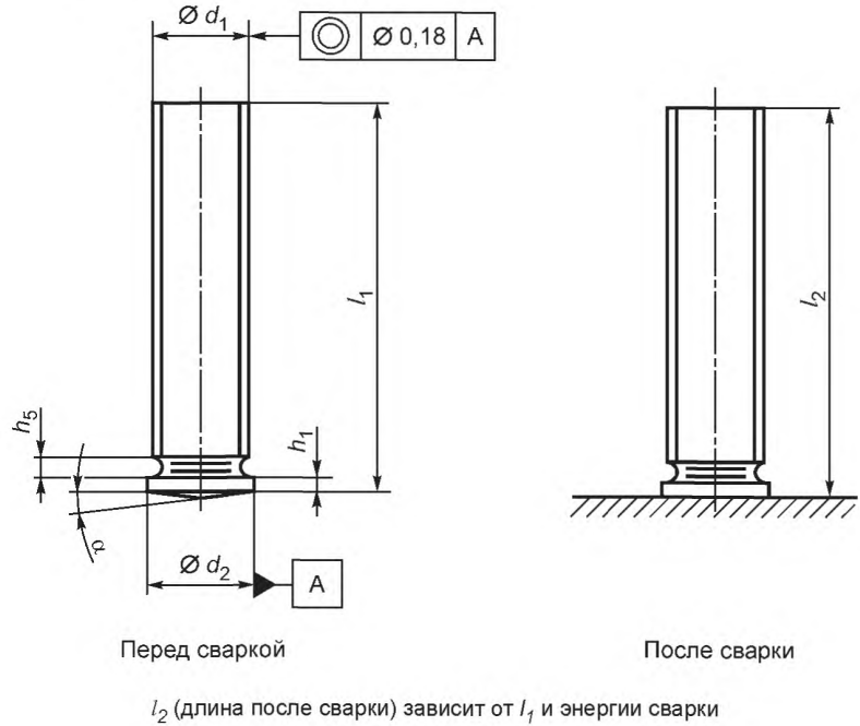
Рисунок 6 — Шпилька с резьбой с фланцем (PS)
