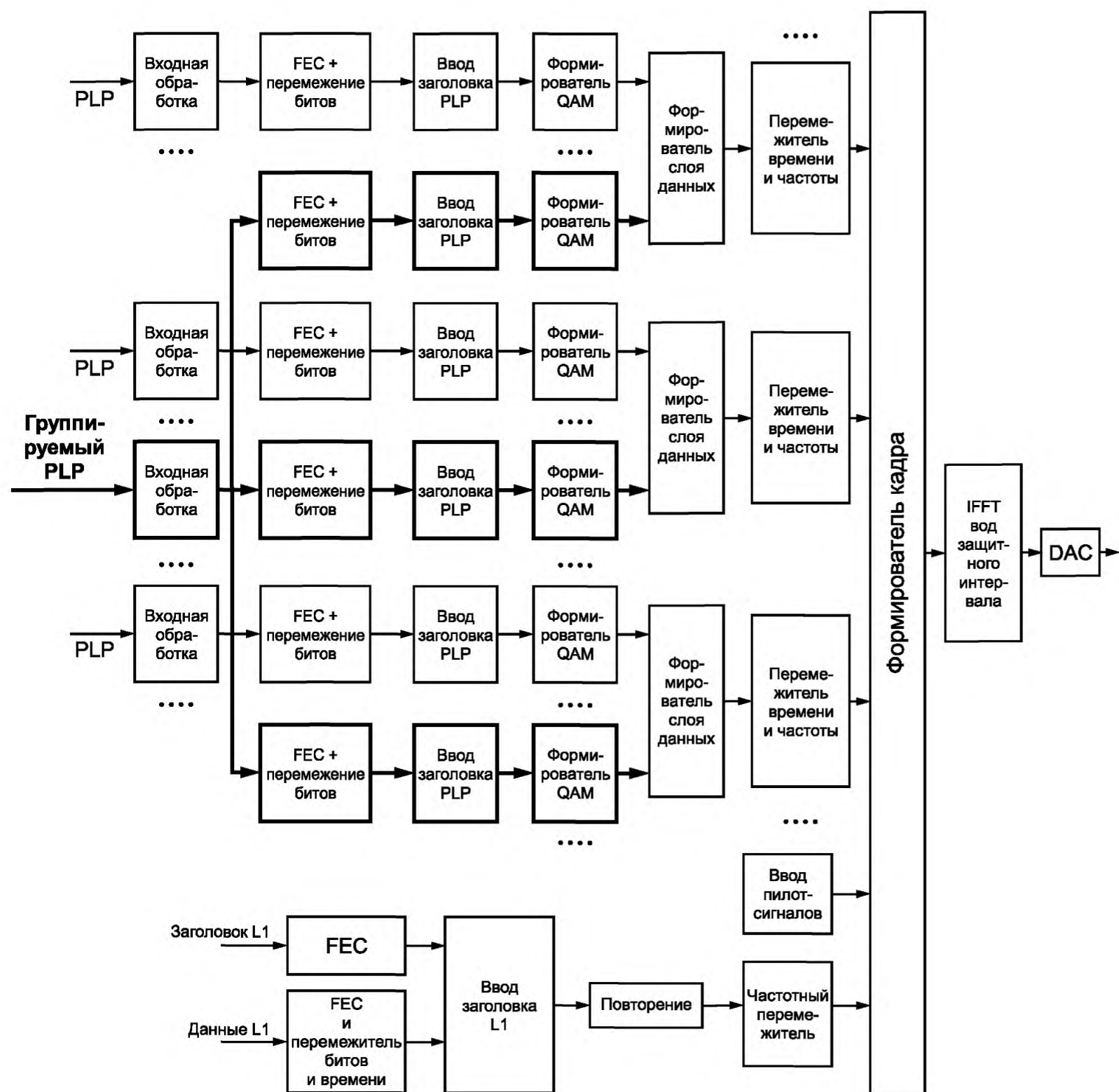
Рисунок Г.1 — Блок-схема режима группирования PLP
