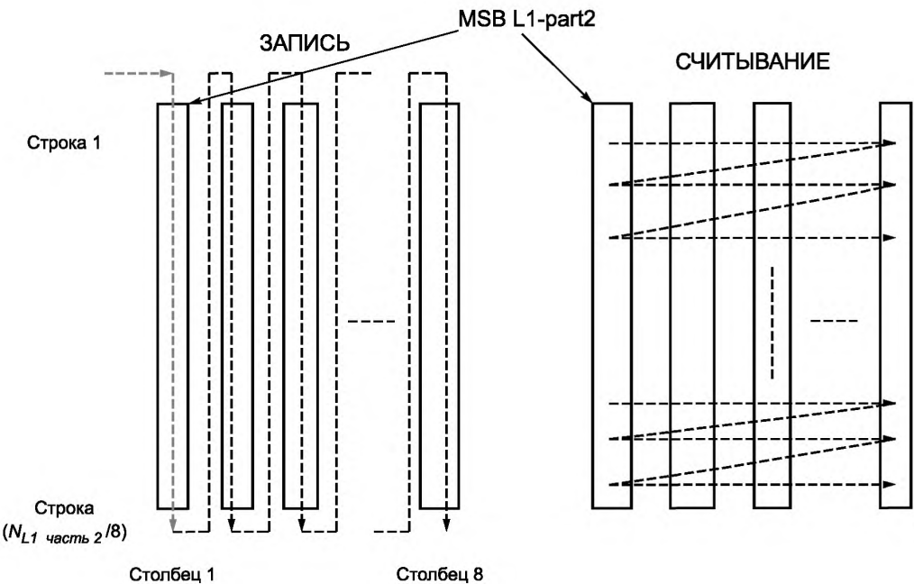
Рисунок 30 — Схема перемежителя битов данных L1-part2 (16QAM)
