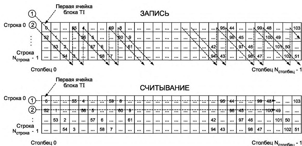
Рисунок 32 — Перемеживание времени данных сигнализации L1 ( N_{MOD\_TOTAL} = 208 , N_{L1\_TI\_DEPTH} = 4 )
