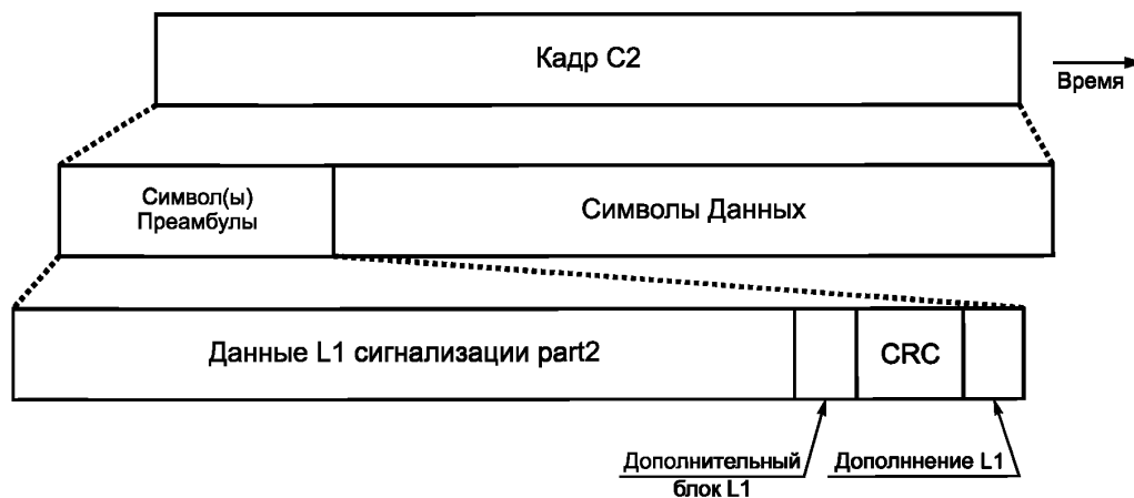
Рисунок 22 — Структура данных сигнализации L1-part2
