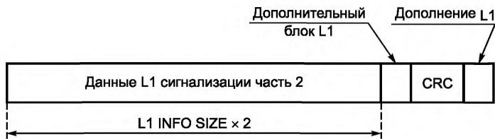
Рисунок 24 — Размер поля L1_INFO_SIZE
