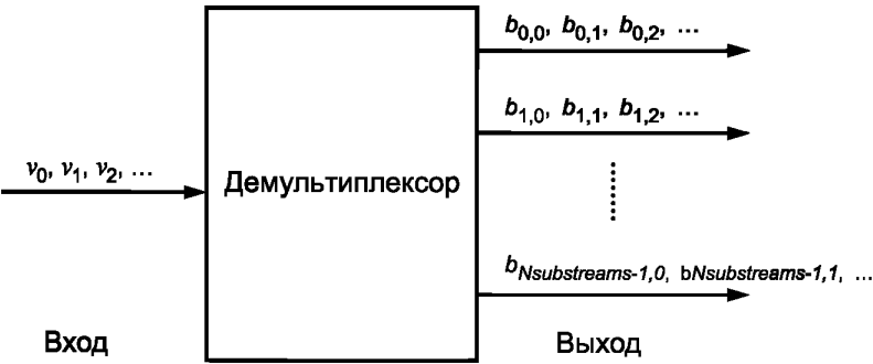
Рисунок 16 — Демультимплексирование битов в субпотoki
