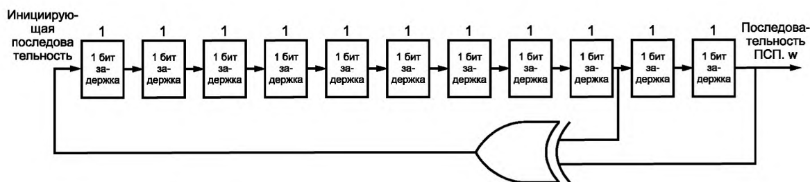
Рисунок 34 — Формирование псевдослучайной последовательности
