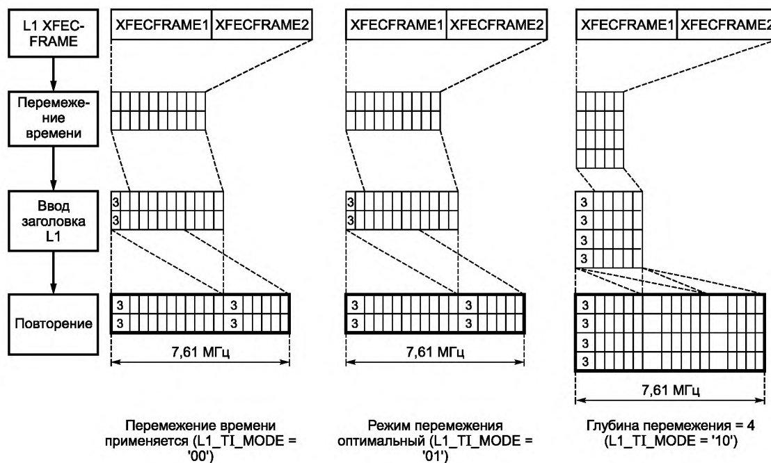
Рисунок 31 — Перемежение времени данных сигнализации L1-part2
