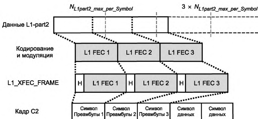
Рисунок 27 — Длина кодированных данных
