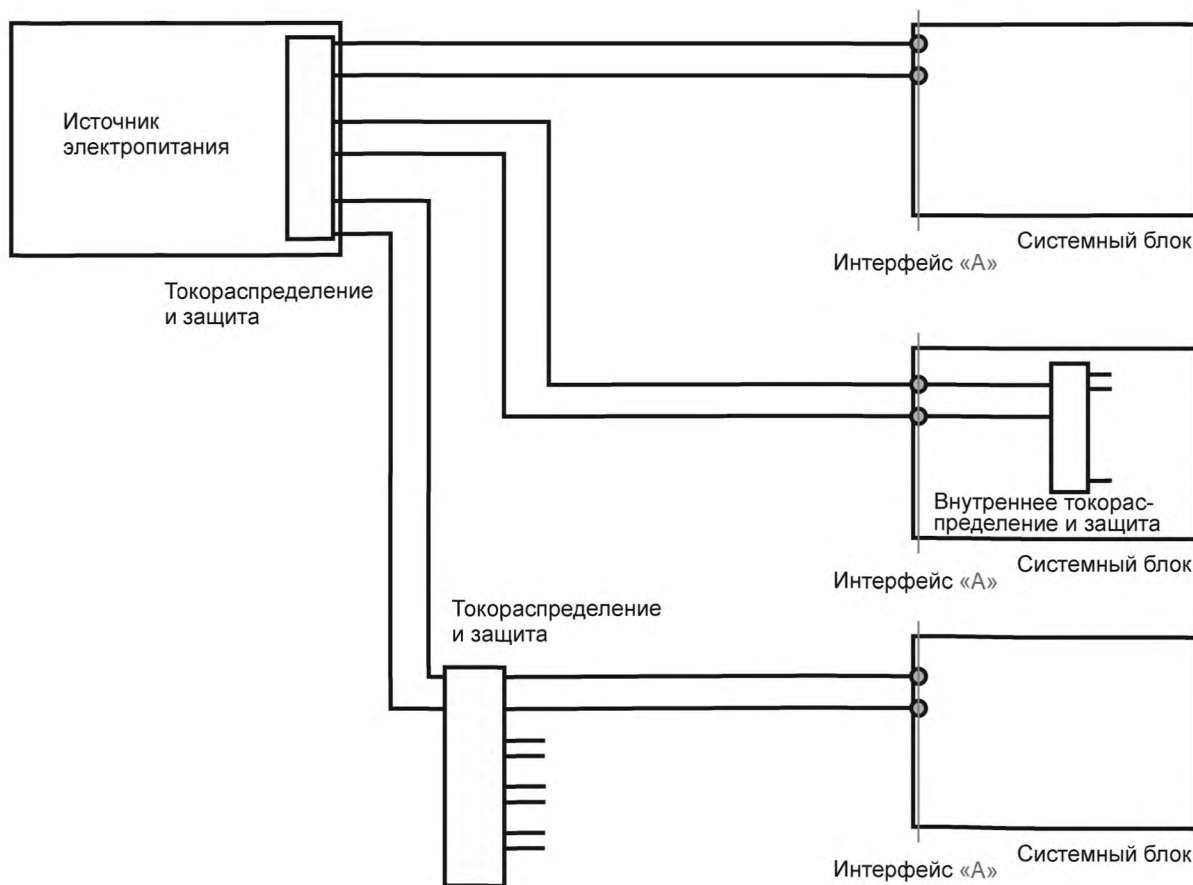
Рисунок Б.1 — Идентификация интерфейса «А»
