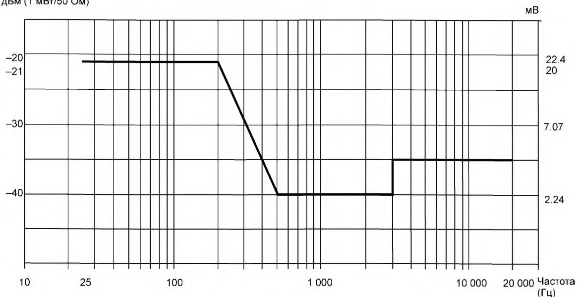
Рисунок 6 — Максимальные уровни узкополосного шума
