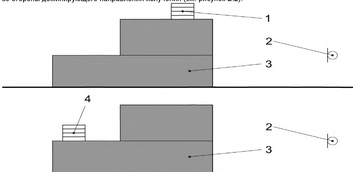
1 – предпочтительное место расположения образцового источника шума; 2 – место установки микрофона; 3 – испытываемый источник шума; 4 – нежелательное место расположения образцового источника шума
