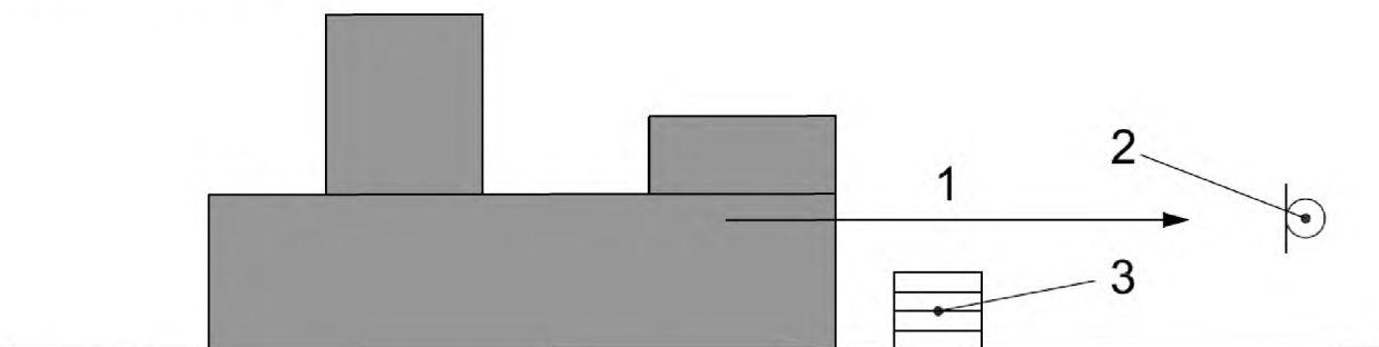
1 – доминирующее направление излучения испытуемого источника; 2 – место установки микрофона; 3 – предпочтительное место расположения образцового источника шума
