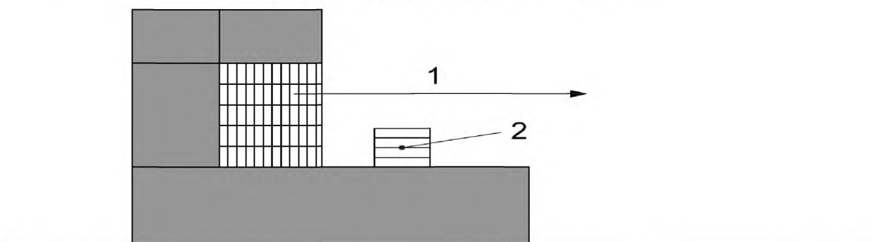
1 – направление доминирующего излучения; 2 – предпочтительное место установки образцового источника шума
