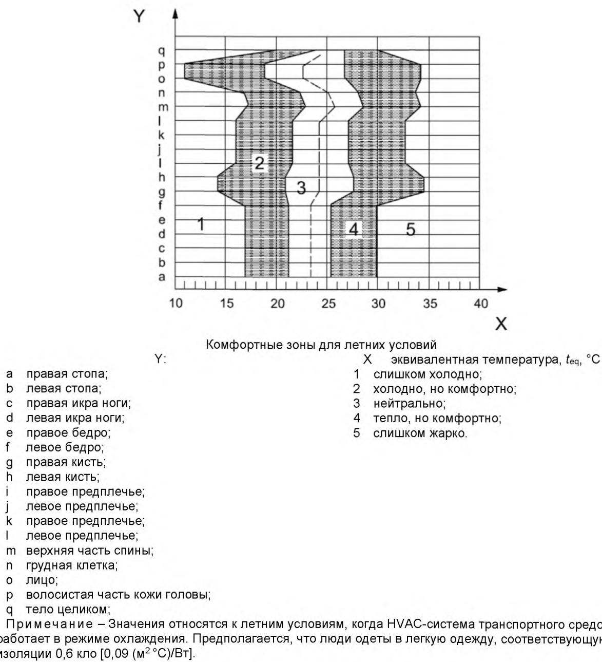
Рисунок D.1 – Предлагаемая схема оценки измеренных значений t_{eq} с позиций субъективного восприятия условий водителем или пассажиром
