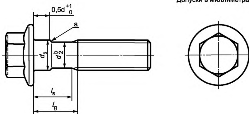
Рисунок 1 — Болт с шестигранной головкой с фланцем — нормальный стержень — стандартный тип
