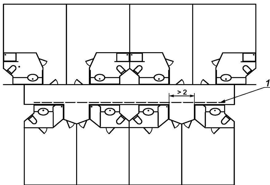
Рисунок F.1 — Расположение световых полос для коридорной ниши
