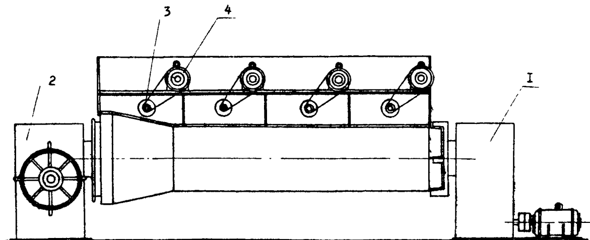
Рис. 17. Схема машины для нанесения защитного слоя.
