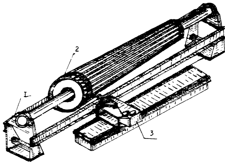
Рис.6. Процесс наливки на станке продольной арматуры. 1 - опорная рама станка; 2 - стержень-катушка, 3 - подвижная каретка.
