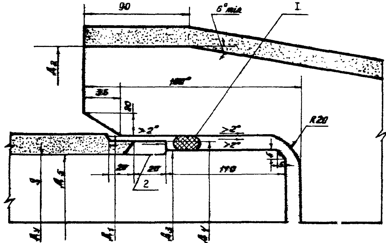
Рис. 1б. Основные размеры раструбов и втулочных концов сердечников труб.
