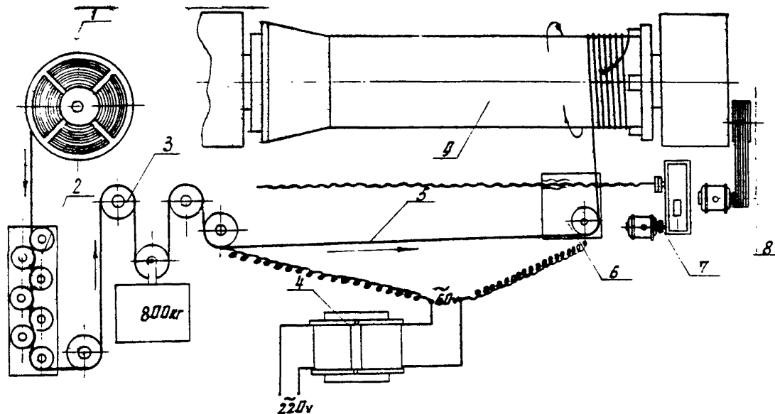
Рис. 15. Машина для намотки предварительно напряженной спиральной арматуры. 1 - бобина-бухтодержатель, 2 - правильно-тормозное устройство, 3 - пост механического натяжения, 4 - трансформатор сварочный, 5 - участок электронного нагрева проволоки, 6 - катетка, 7 - привод ходового винта катетки, 8 - привод ведущей бочки, 9 - навиваемый сердечник трубы.
