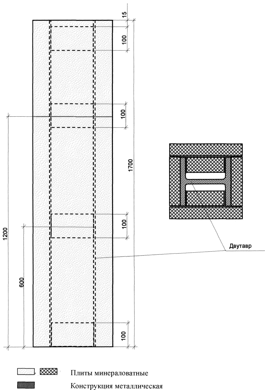
Рисунок 5.3 – Пример расположения плит и вставок на двутавре
