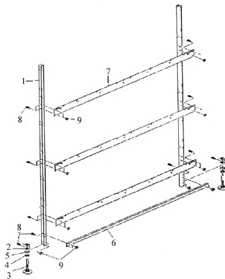
Рисунок 3 – Сборка щита (первый этап)
