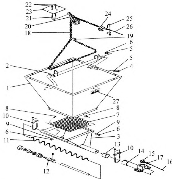
Рисунок 42 – Схема монтажа верхней части к нижней части бункера корма
