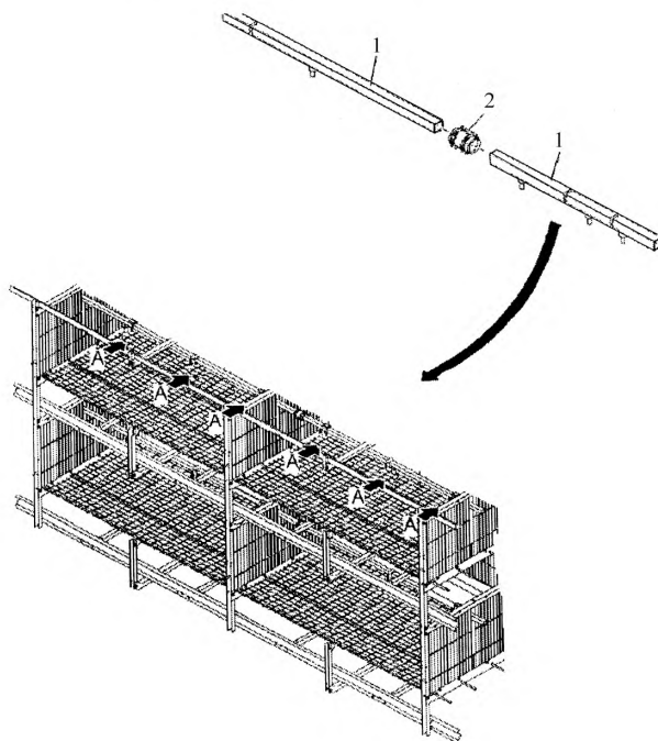
Рисунок 23 – Узлы для монтажа системы поения
