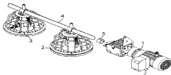
Рисунок 28 – Узлы привода
