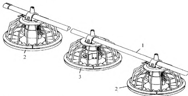
1 – концевая труба; 2 – кормушка; 3 – контрольная кормушка
