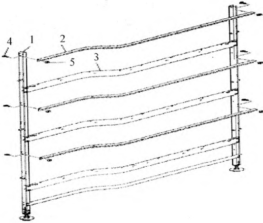
Рисунок 4 – Сборка щита (второй этап)
