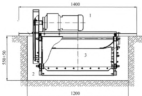
1 – привод; 2 – канал; 3 – пометоуборочный транспортер
