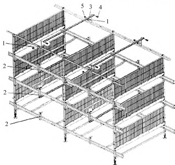
Рисунок 9 – Сборочные узлы и детали для монтажа кронштейнов
