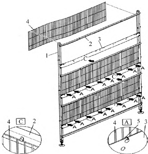
Рисунок 5 – Сборка щита (третий этап)
