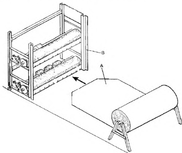
Рисунок 32 – Схема заправки пометоуборочной ленты вручную
