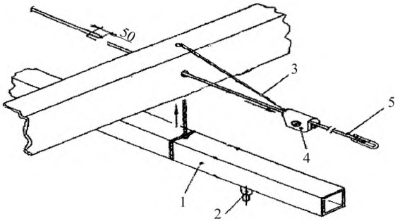
1 – трубопровод для подачи воды; 2 – ниппель; 3 – трос диаметром 1 мм; 4 – хомут пластиковый; 5 – трос Рисунок 25 – Узел подвеса системы поения в сборке
