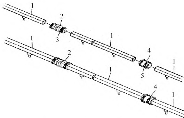
Рисунок 23 – Узлы для монтажа системы поения
