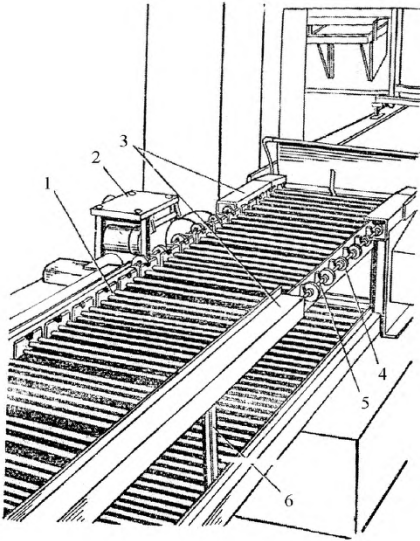
Рисунок 54 – Транспортёр ТСЯ-20.
