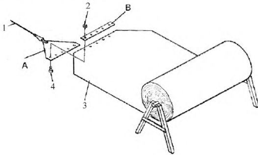
Рисунок 33 – Схема заправки пометуюборочной ленты при помощи натяжного троса
