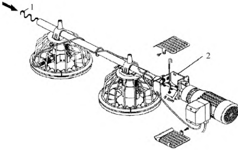
Рисунок 29 – Узлы гибкого шнека
