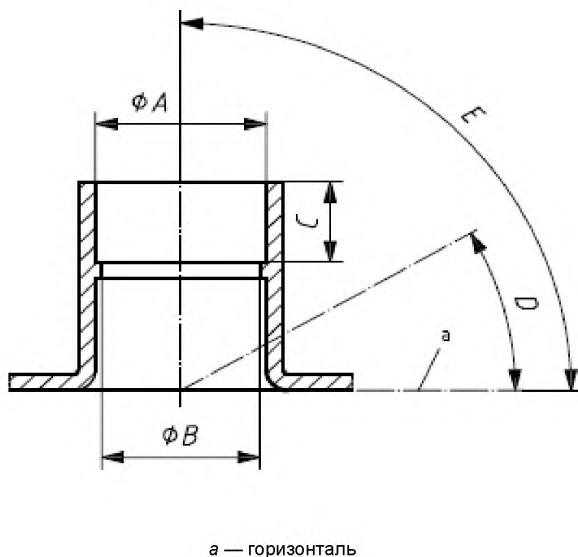
Рисунок 1 — Заливная горловина
