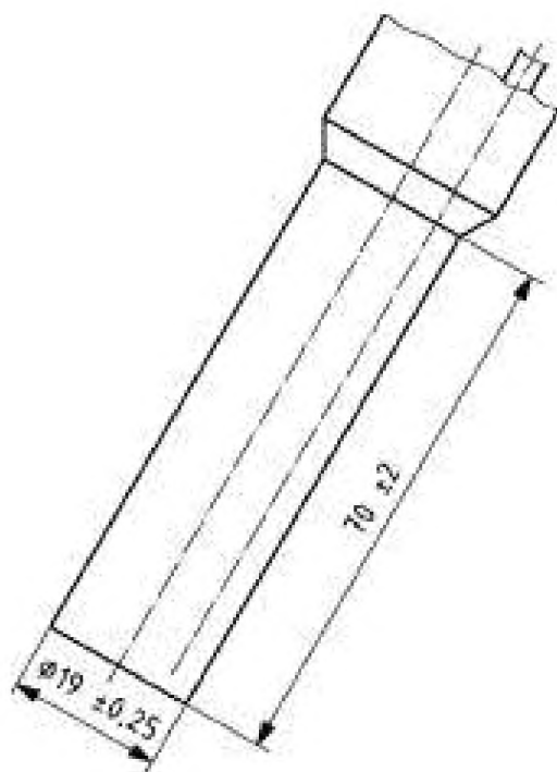
Рисунок 3 — Сопло
