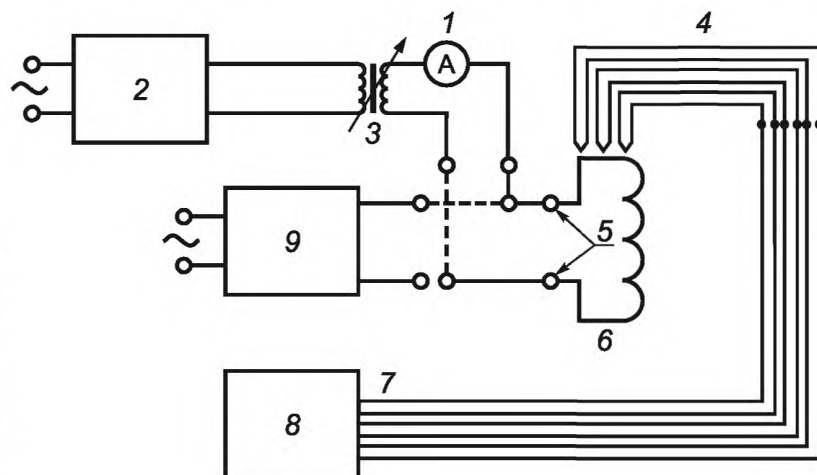
Рисунок 4 — Схема расположения основного и дополнительного оборудования
