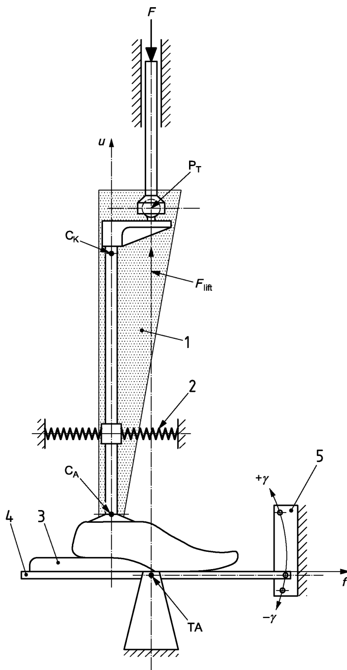
Рисунок 8 – Схематическое изображение испытательного оборудования с испытываемым образцом
