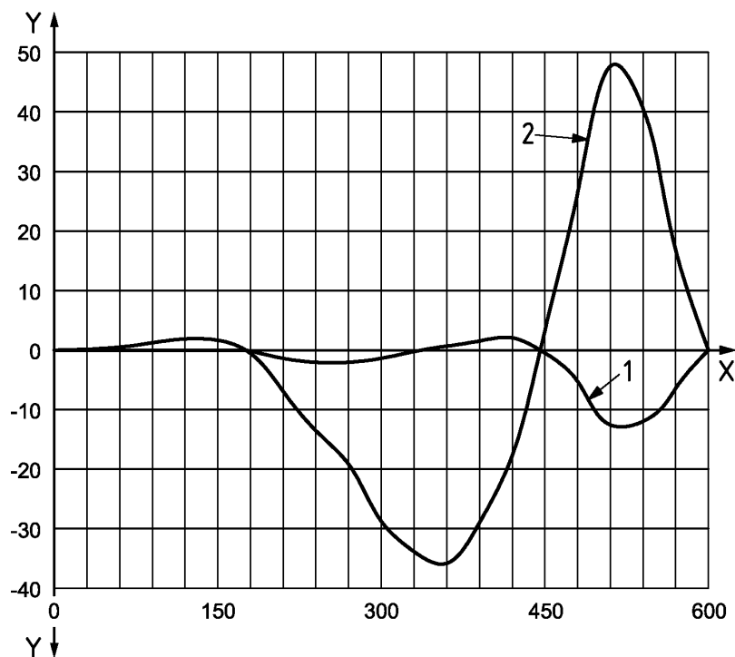
Рисунок 16 – Иллюстрация отклонения сил, воспроизводимых кривошипно-шатунным механизмом 60:40
