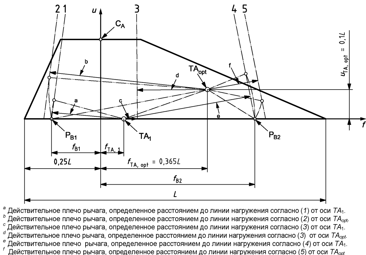
Рисунок 25 – Иллюстрация действительных плеч рычагов
