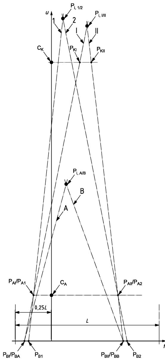
Рисунок 4 – Иллюстрация различных условий нагружения при уровне нагрузки P_5
