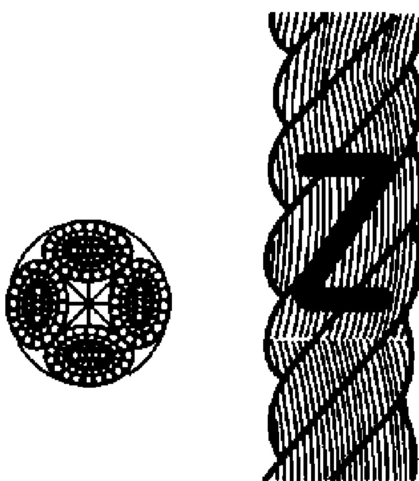
Рисунок 2- Конфигурация 4-рядного крученого каната (тип В)
