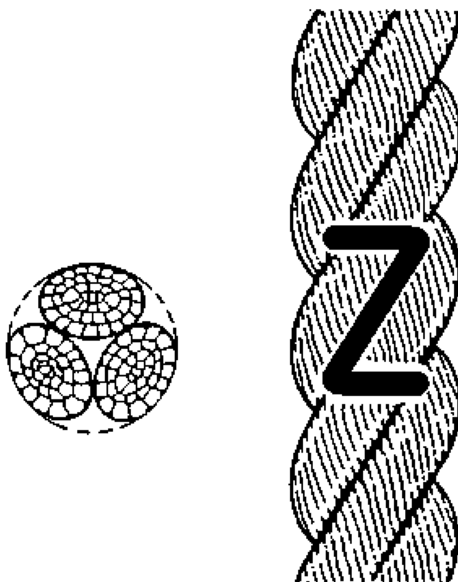
Рисунок 1- Конфигурация 3-рядного крученого каната (тип А)
