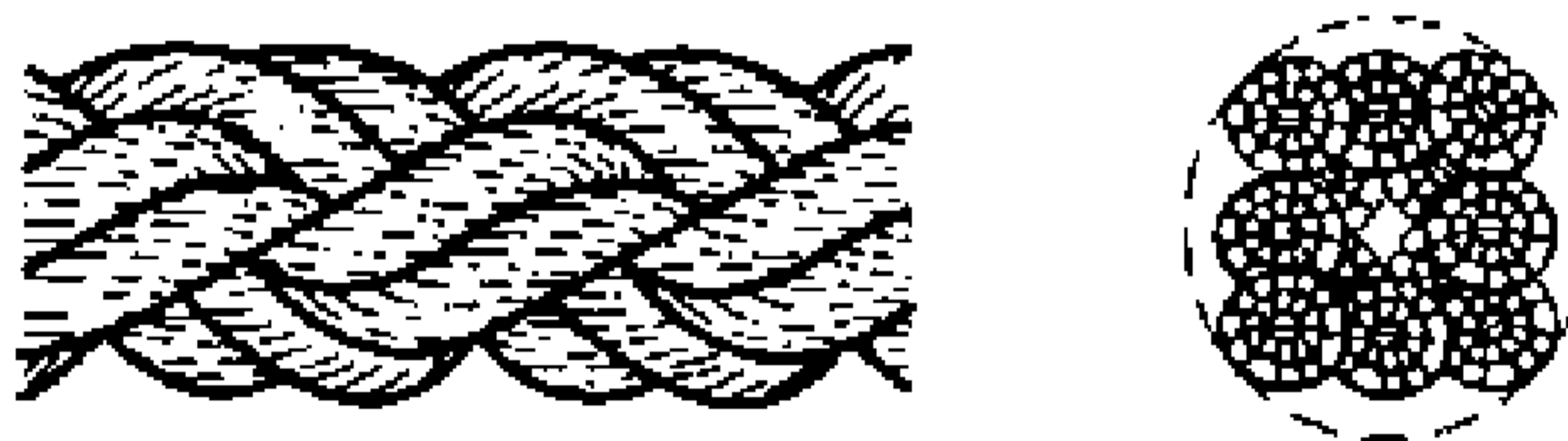
Рисунок 3- Конфигурация 8-рядного плетеного каната (тип L)
