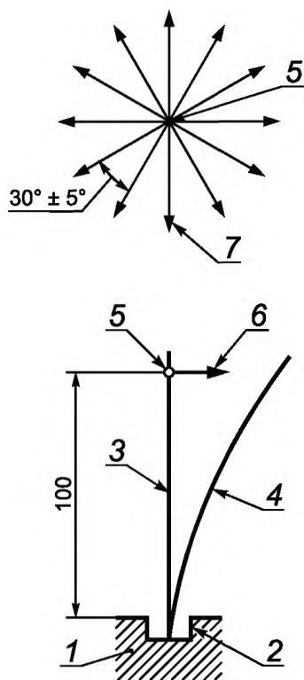
Рисунок 2а) — Принцип устройства установки для испытания на прогиб безвинтовых зажимов
