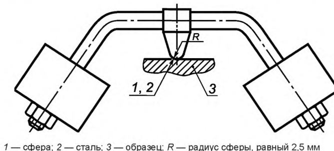
Рисунок 12 — Установка для испытания давлением шарика
